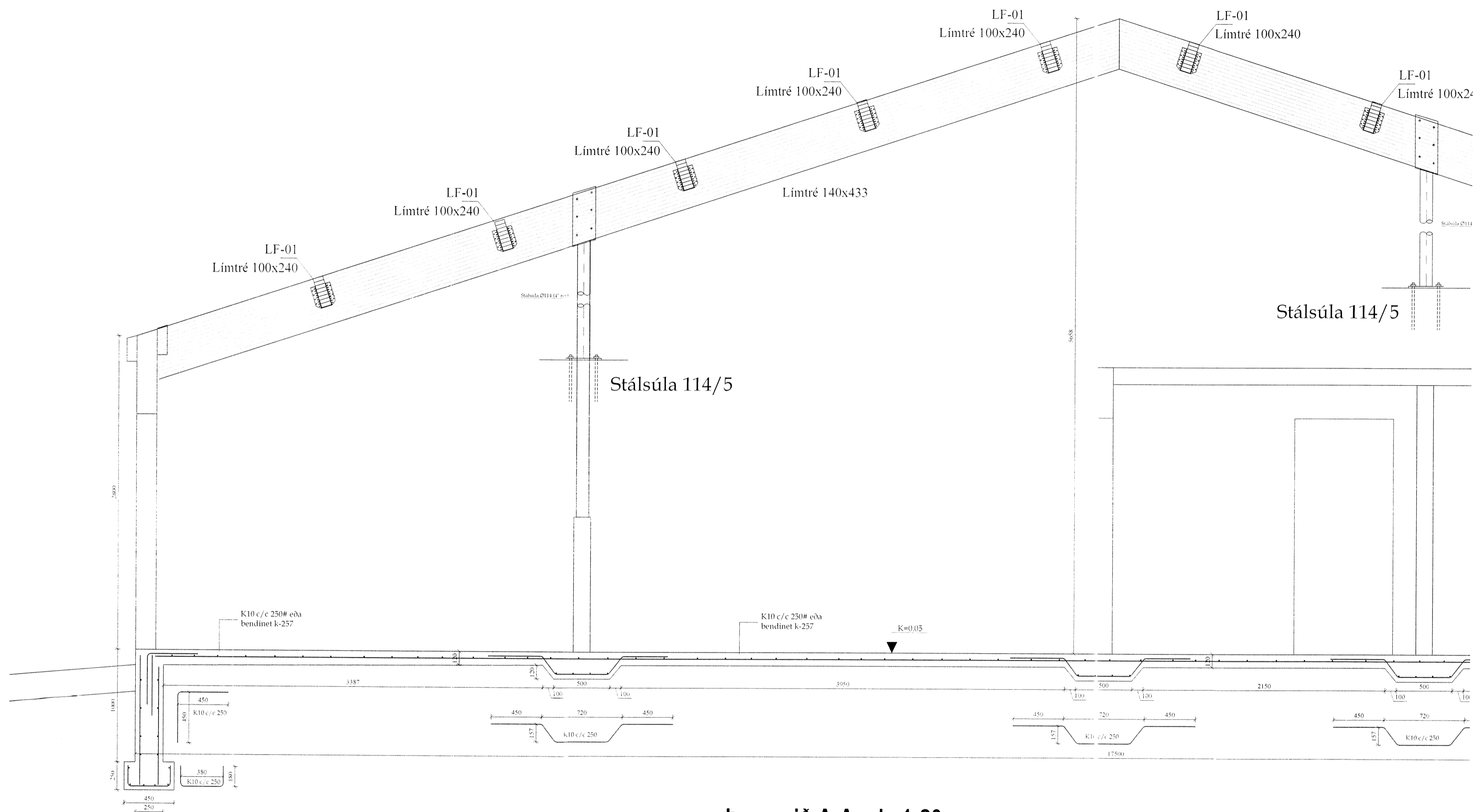
Þversnið A-A mk. 1:20
