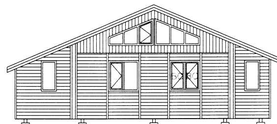
Útlit norður 1:100
