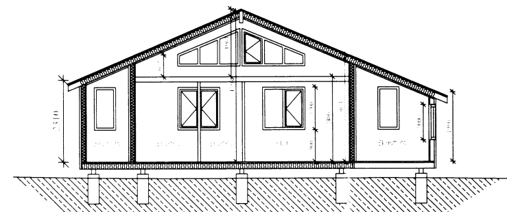
Snið A:A 1:100
