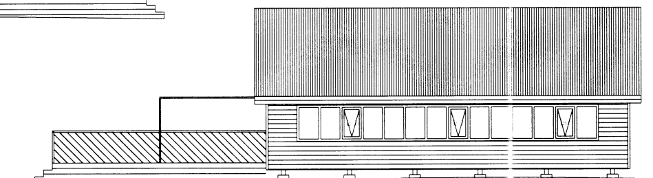
Útlit austur 1:100
