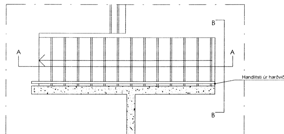
Stigi 1:50
