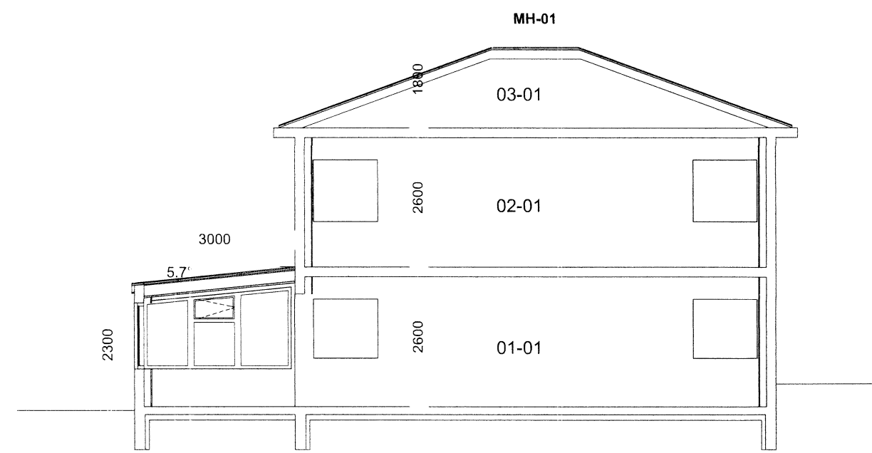
S 1.01 1:100
