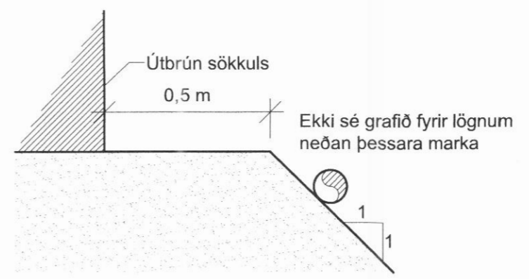
Lega lagna við hús 1:20
