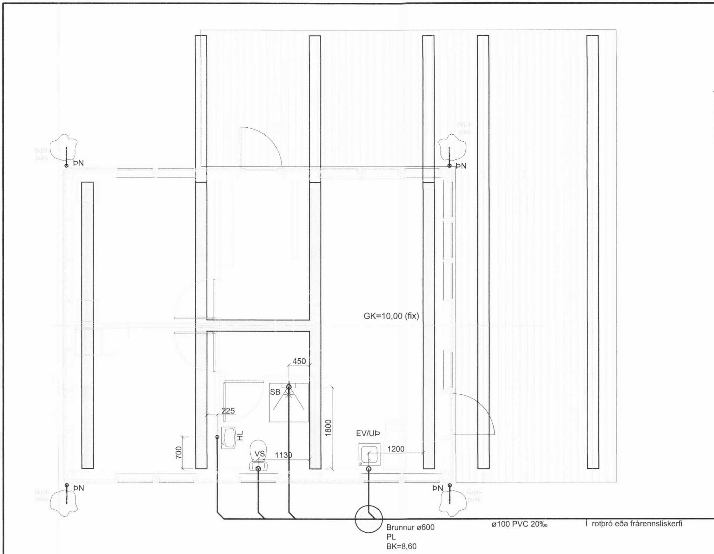
Grunnmynd frárennislagna Mkv. 1:50
