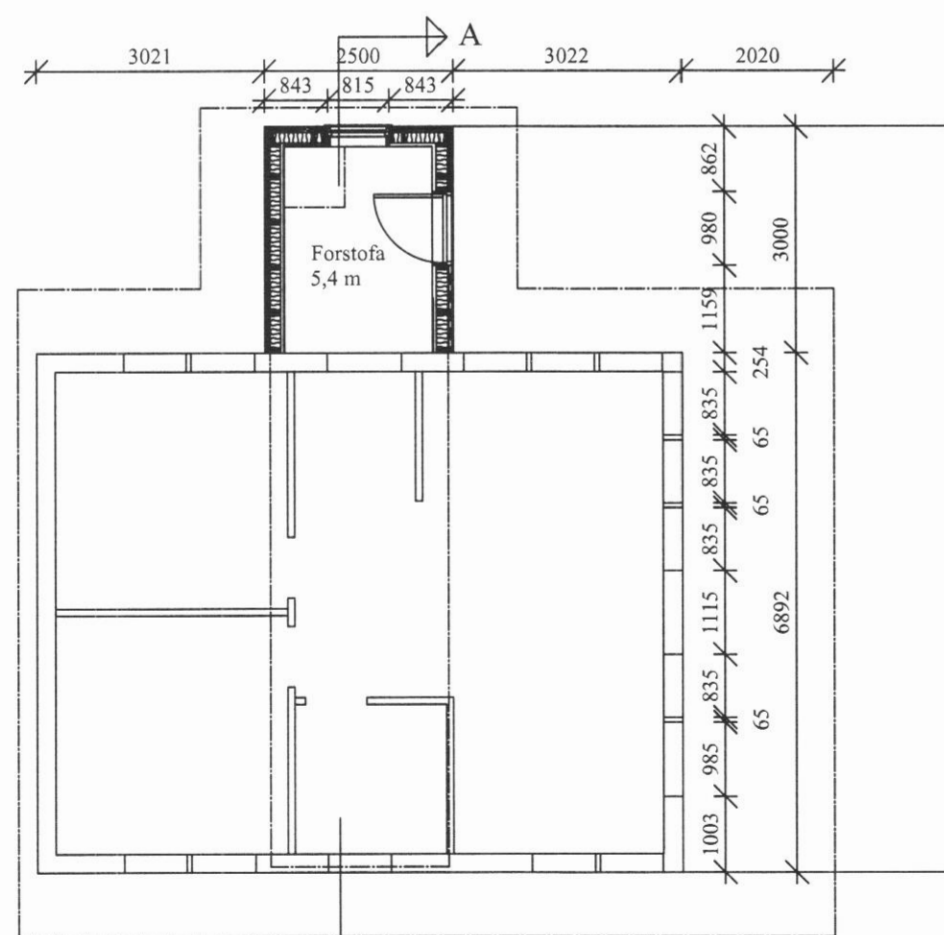
Grunnmynd 1:100
