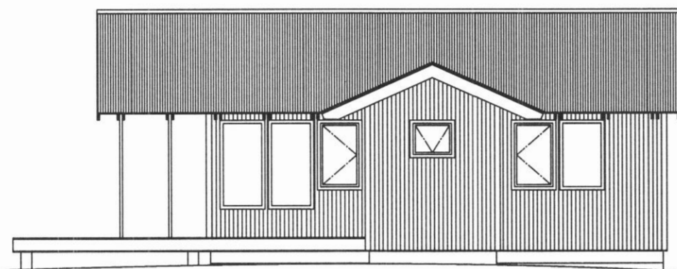
Útlit austur 1:100
