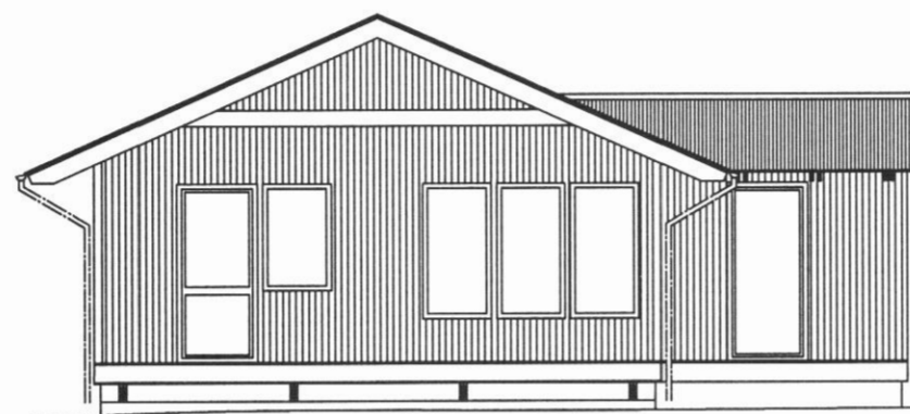
Útlit suður 1:100
