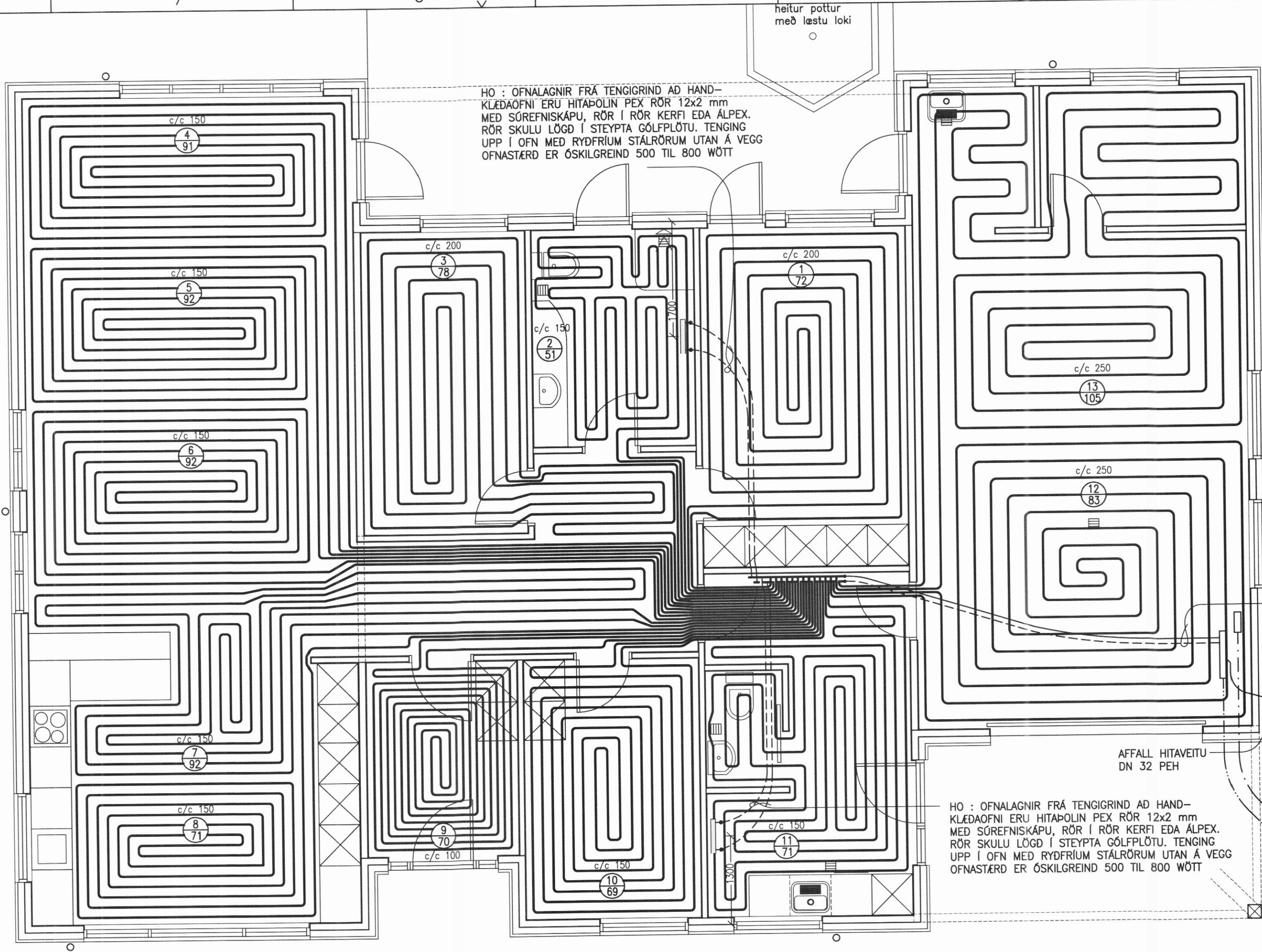
GÓLFHITALAGNIR GRUNNMYND 1:50
