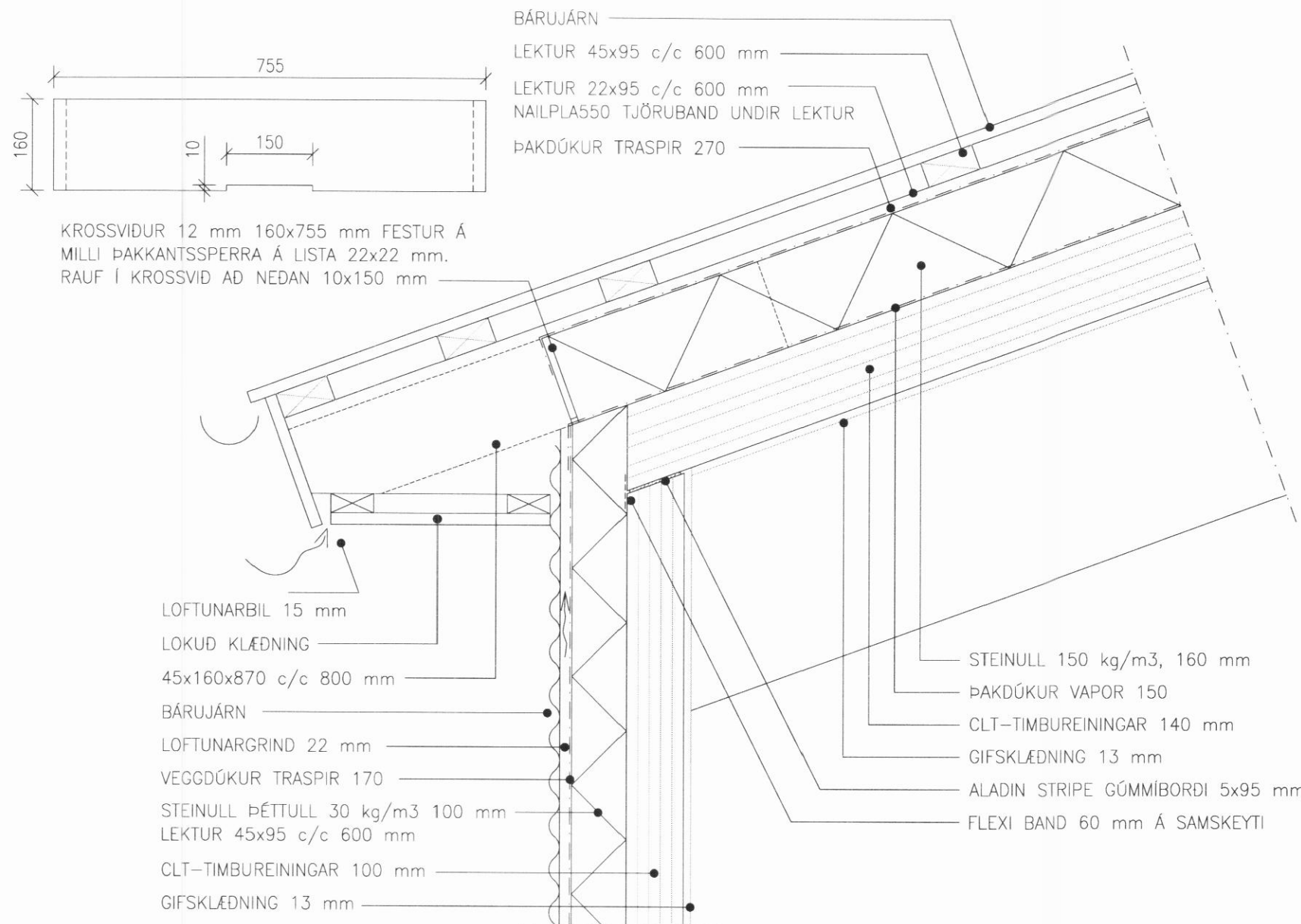
FRÁGANGUR VIÐ ÚTVEGG OG ÞAK 1:10
