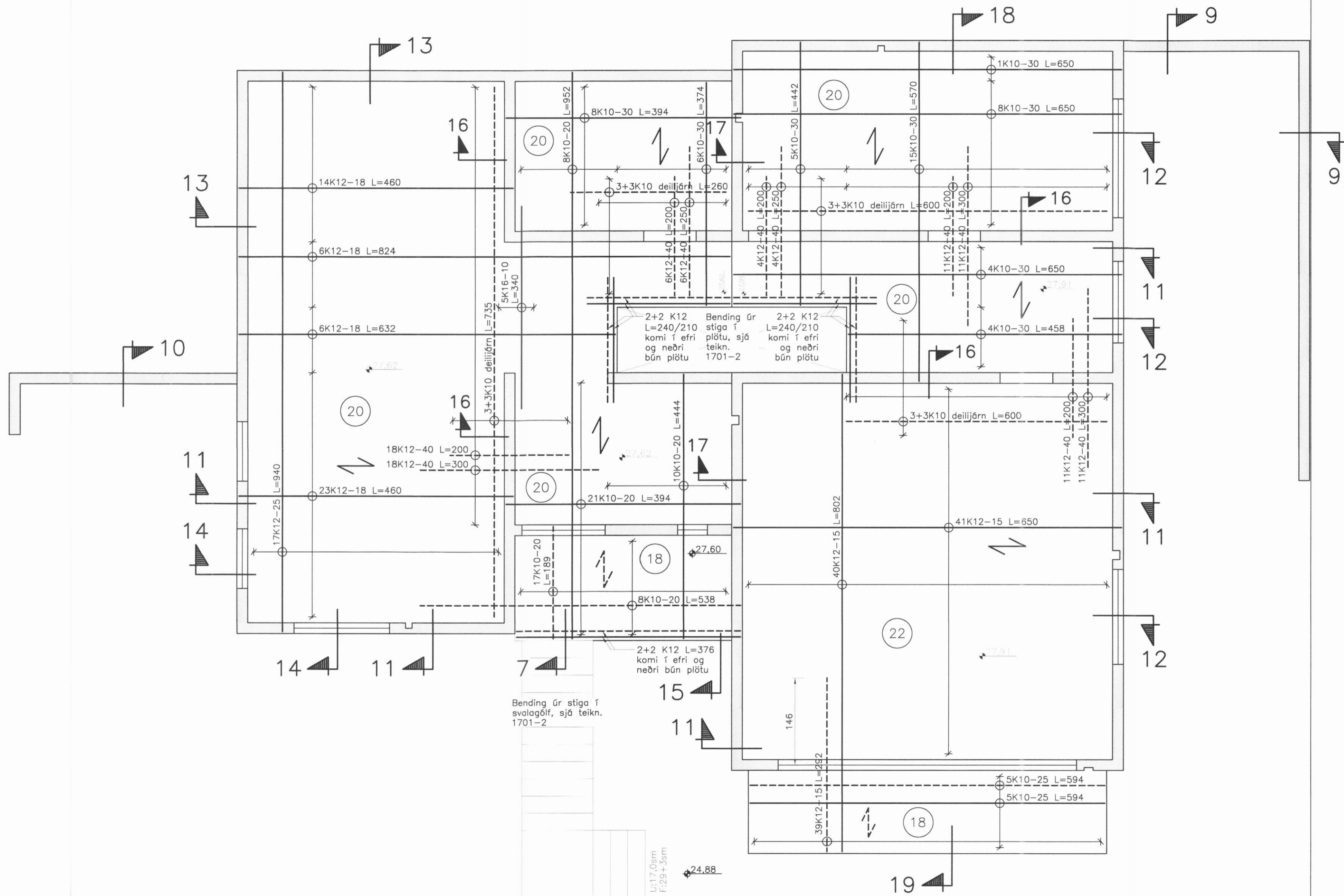
Járn í plötu yfir kjallara 1:50
