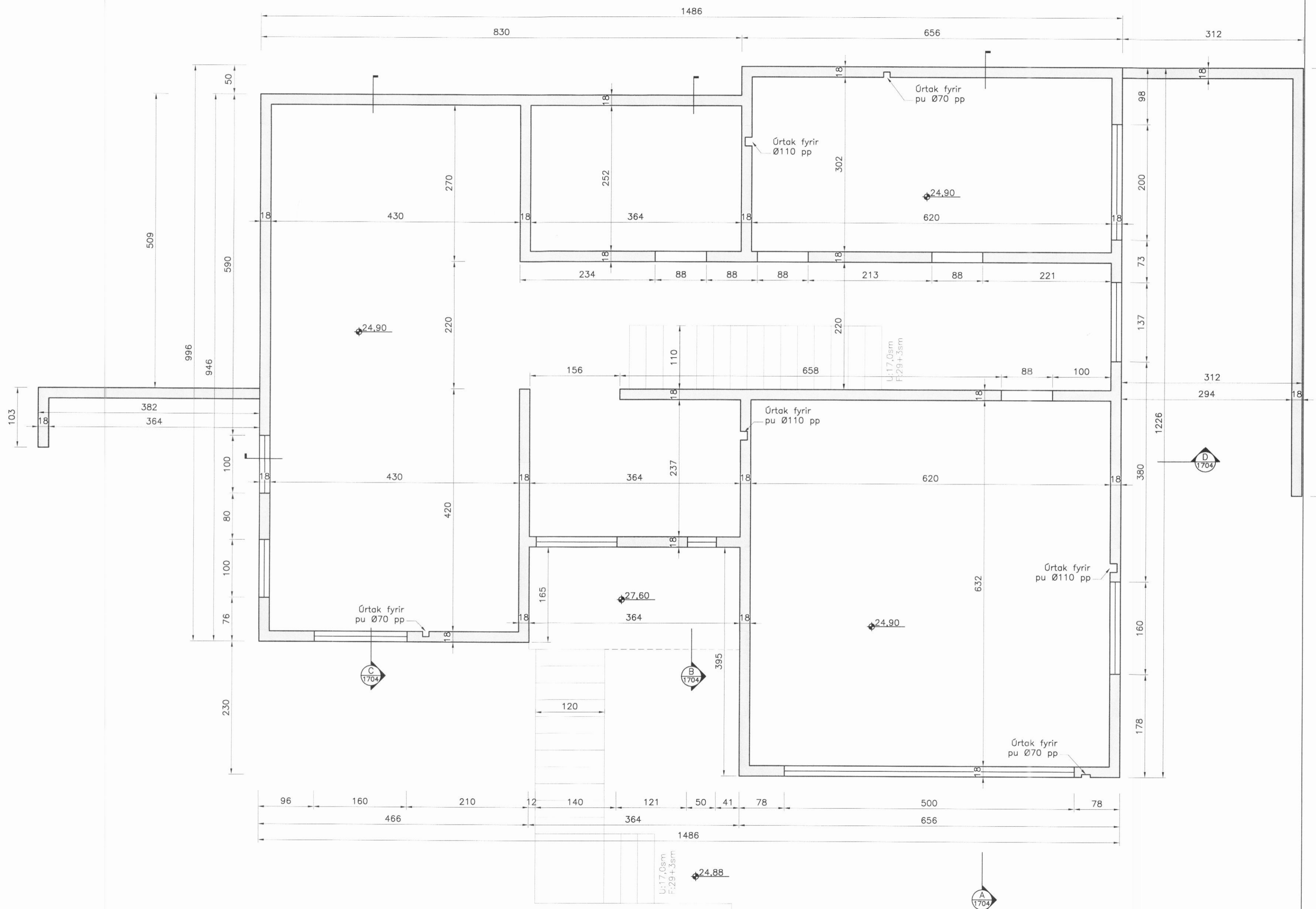
Málsetning steyptra veggja kjallara 1:50
