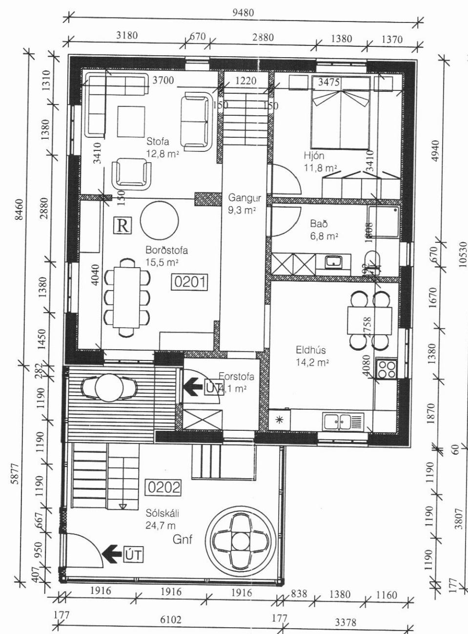
Grunnmynd kjallari 1:100
