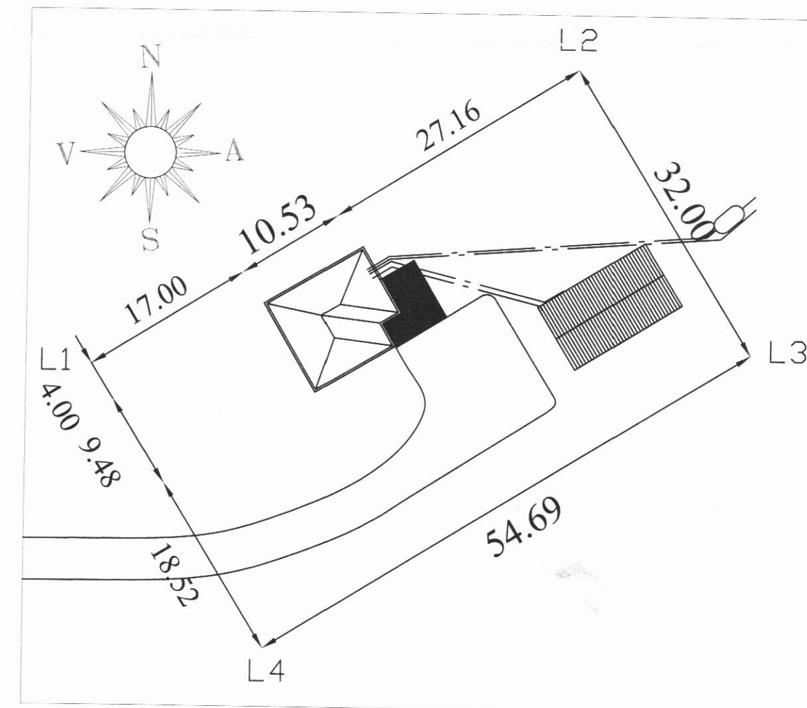
Afstöðumynd 1:500
