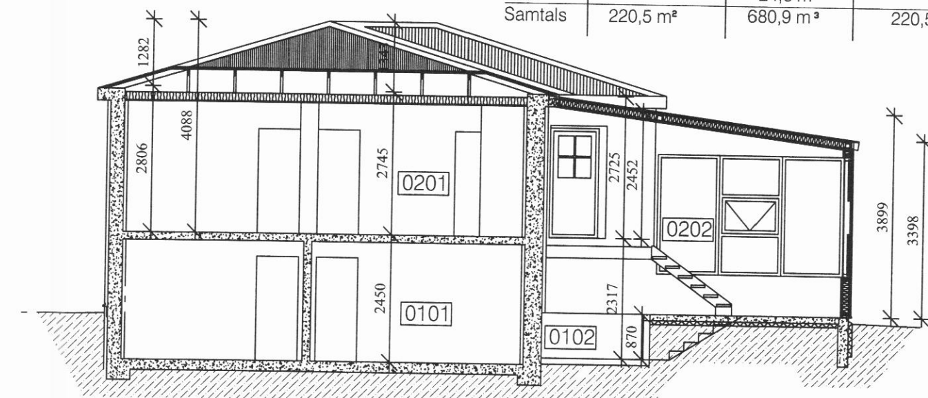
Snið A:A 1:100
