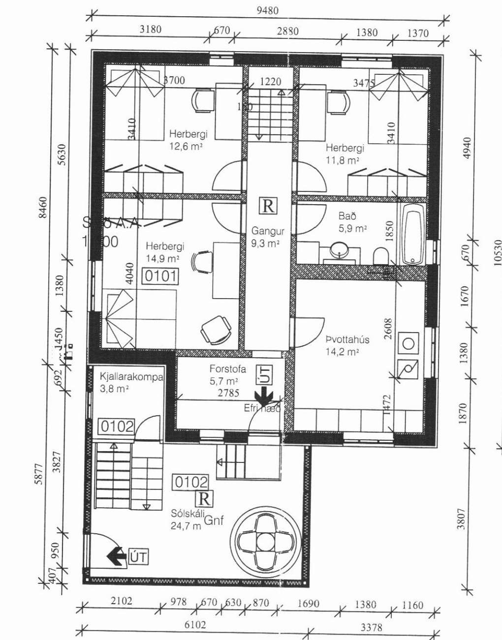
Grunnmynd jarðhæð 1:100
