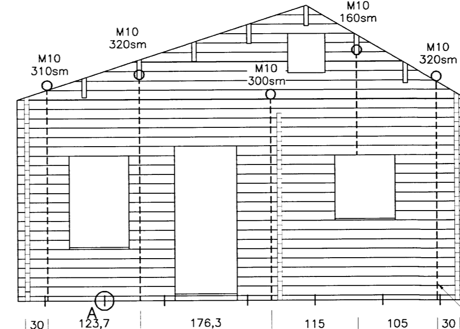
Vesturhlið. Mkv.1:50
