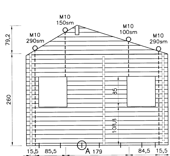
Austurhlið. 1:50
