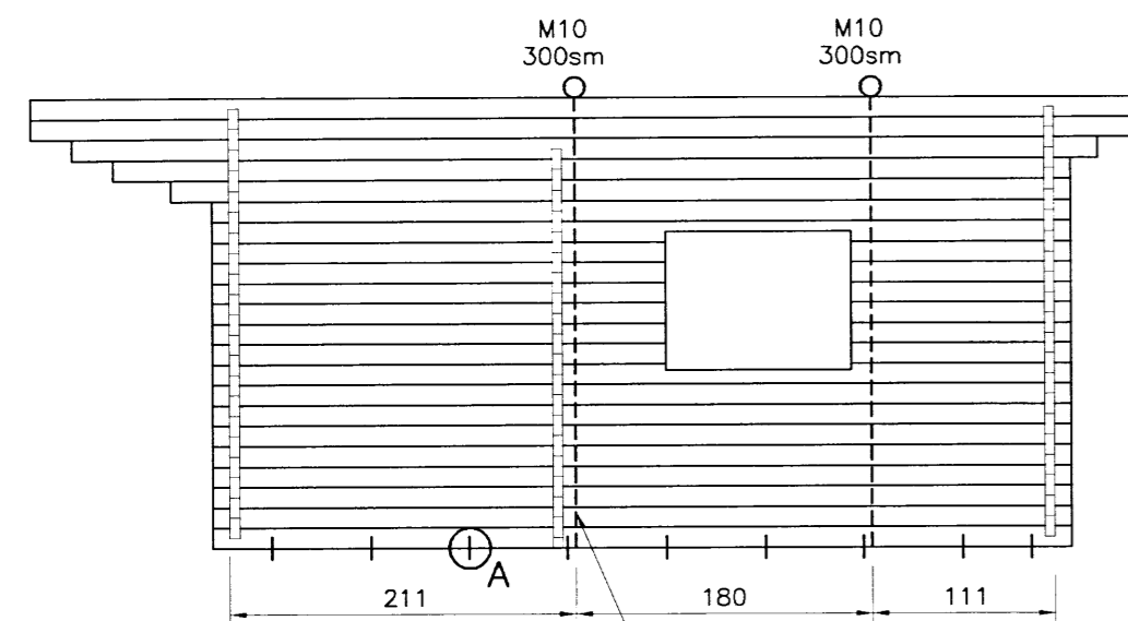
Suðurhlið. Mkv.1:50
