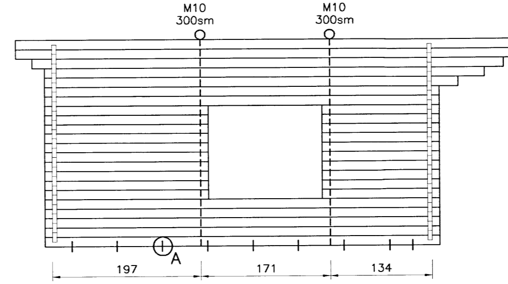
Norðurhlið. Mkv.1:50
