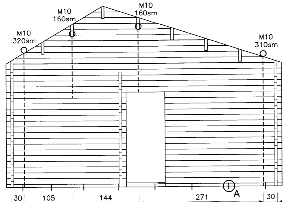
Austurhlið. Mkv.1:50
