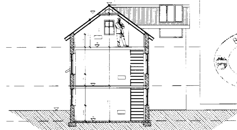
Snið A:A 1:100
