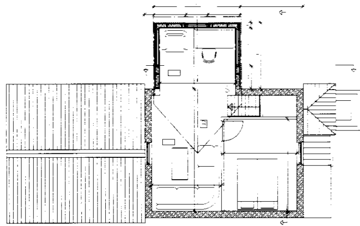
Grunnmynd íshæð 1:100
