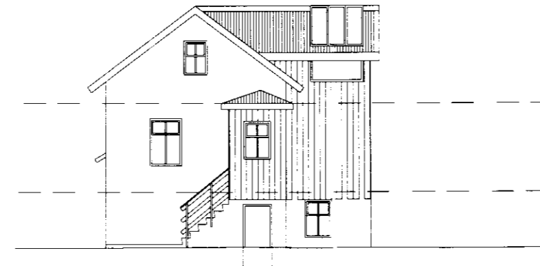
Útlit austur 1:100
