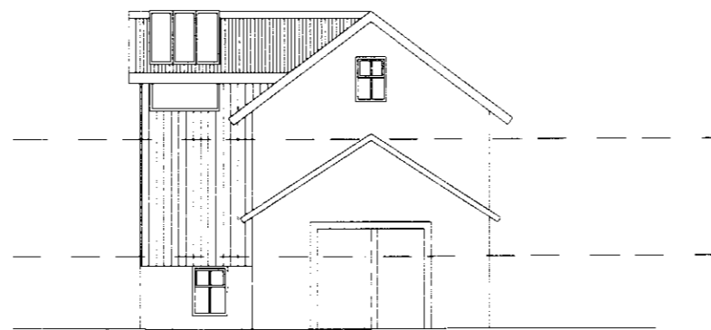
Útlit vestur 1:100
