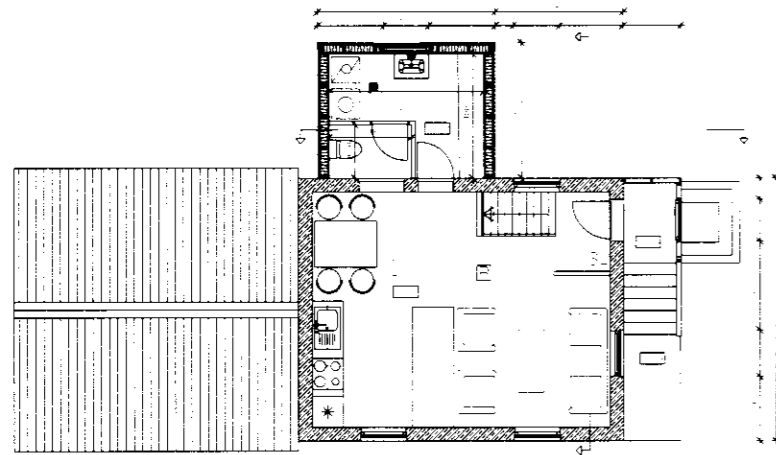
Grunnmynd 1.hæð 1:100
