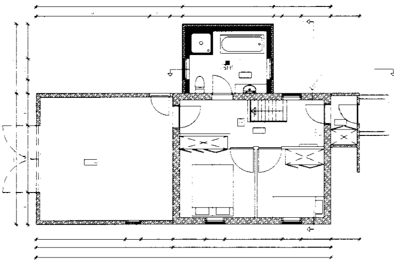
Grunnmynd kjallara 1:100
