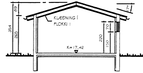
SNÍÐ A-A MKV. 1:100
