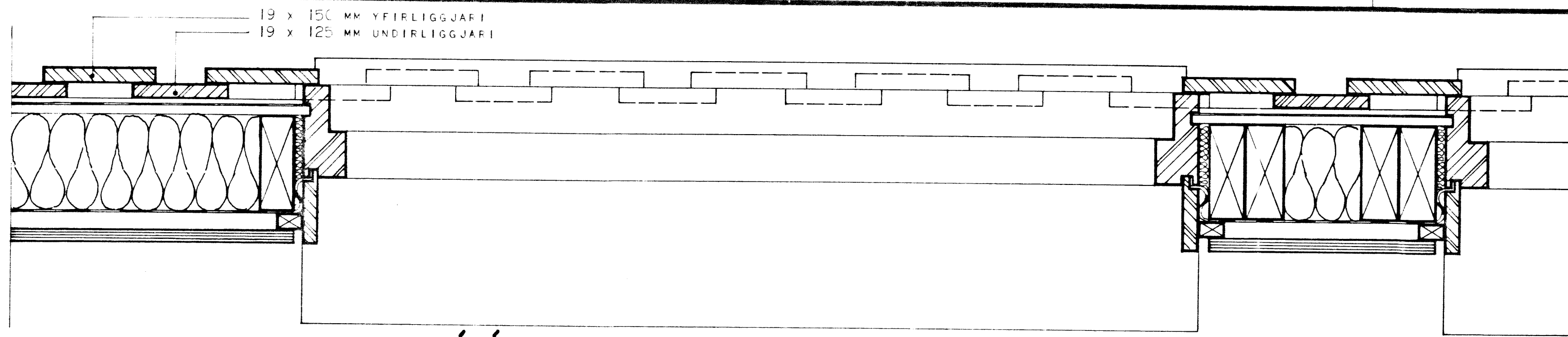
LÁRÉTT SNEIÐING
