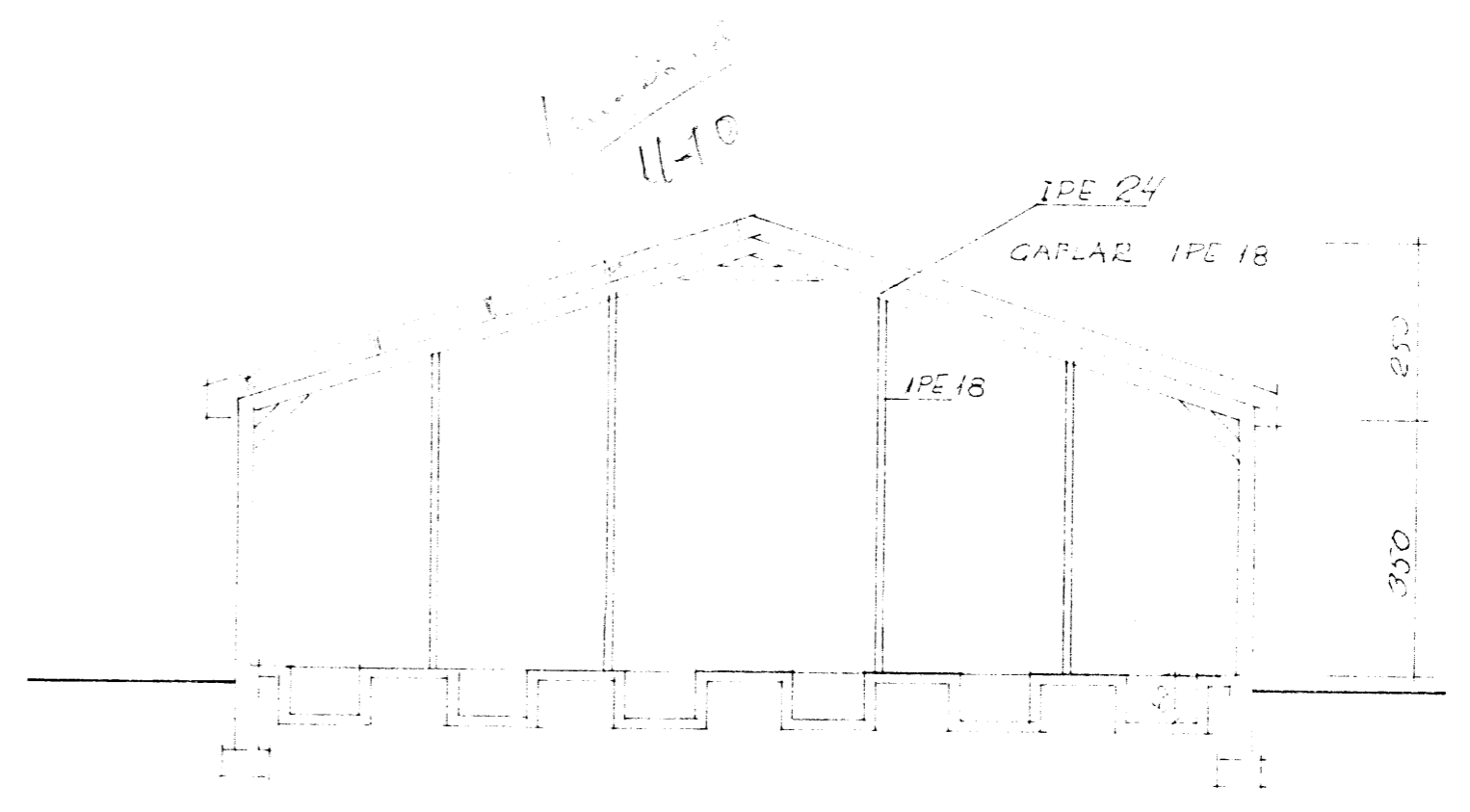
SNID A-A
