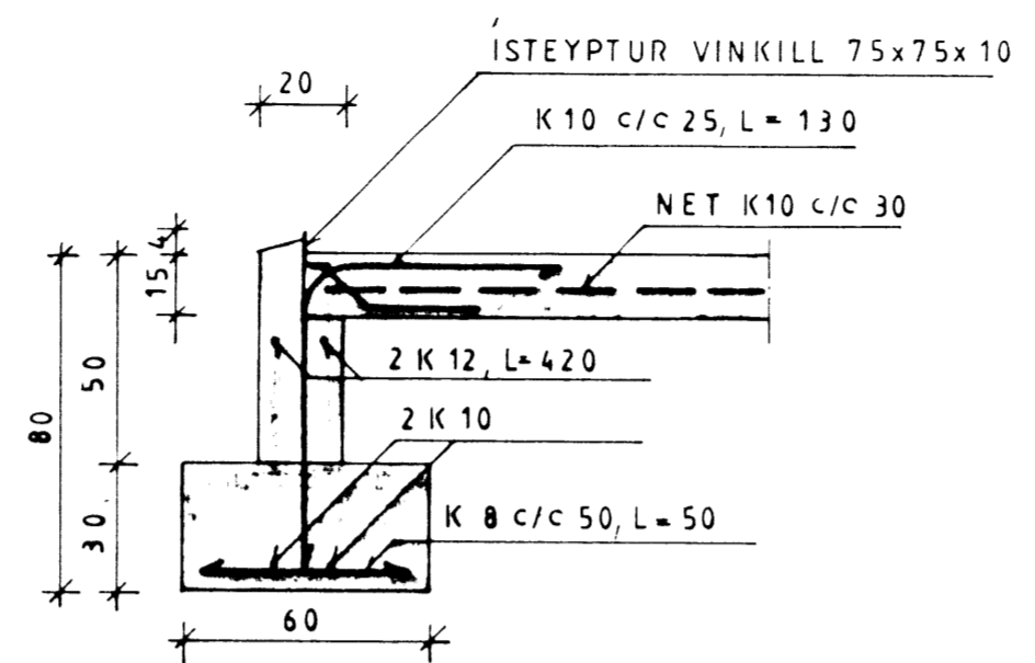
SNID 5-5, 1:20
