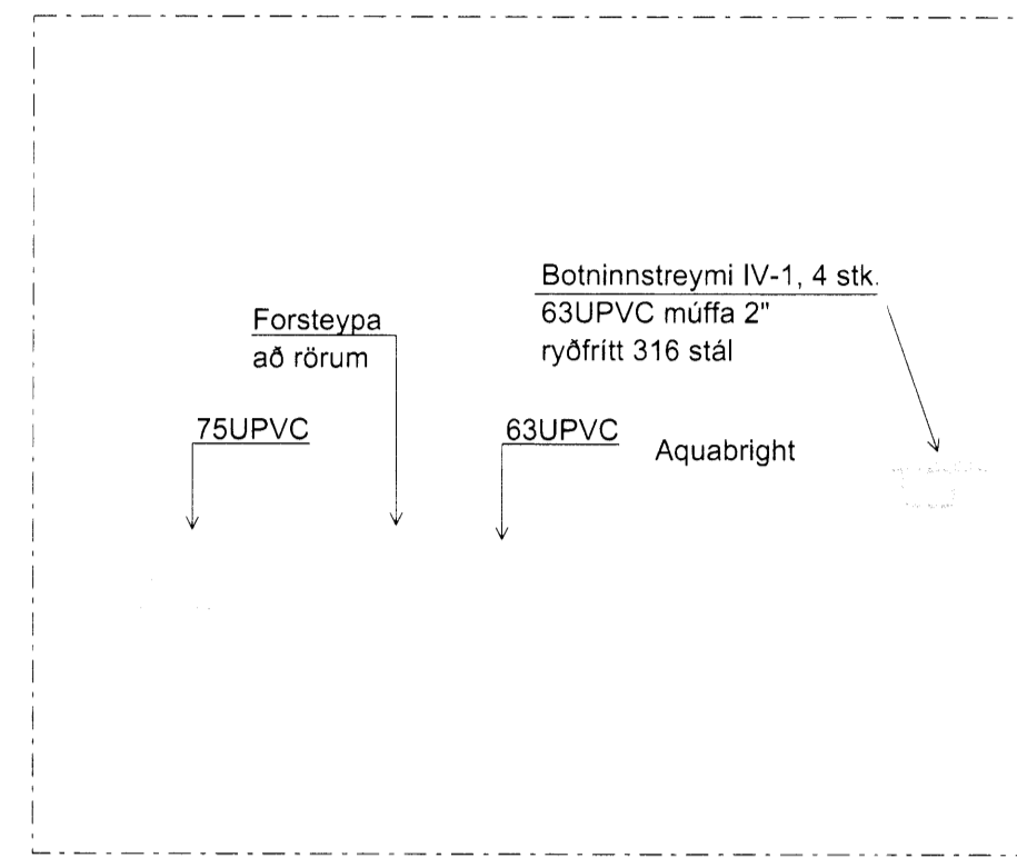
Vaðlaug - botninnstreymi Mkv. 1:10
