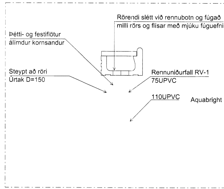
Vaðlaug - rennuniðurfall Mkv. 1:10
