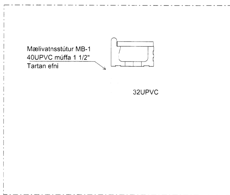
Bláa lónið - mælivatnsstútur Mkv. 1:10
