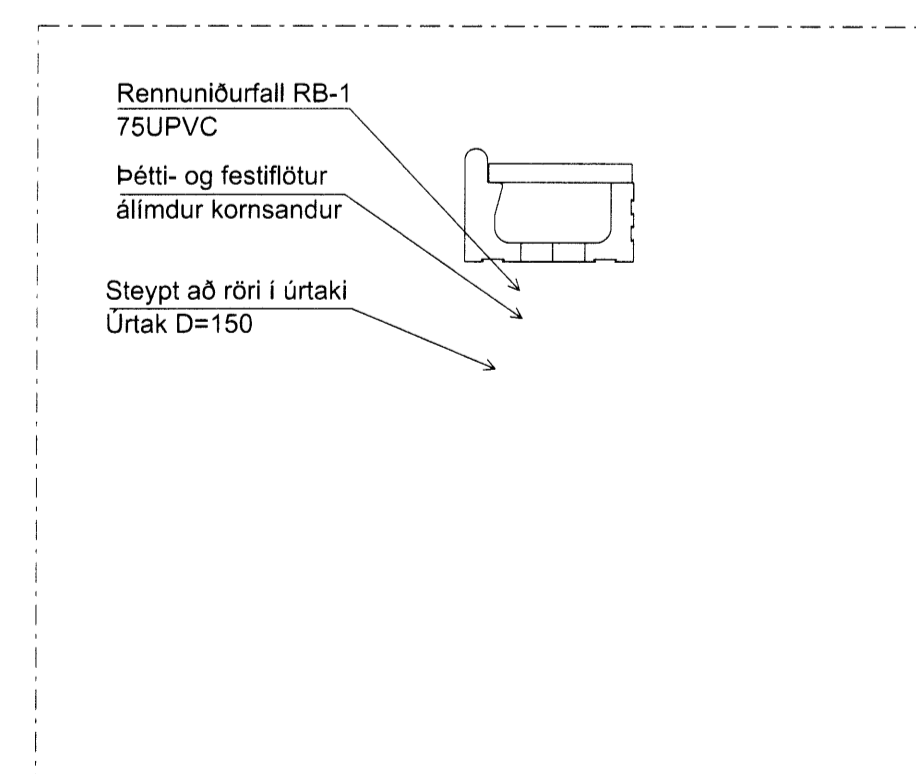
Bláa lónið - rennuniðurfall Mkv. 1:10
