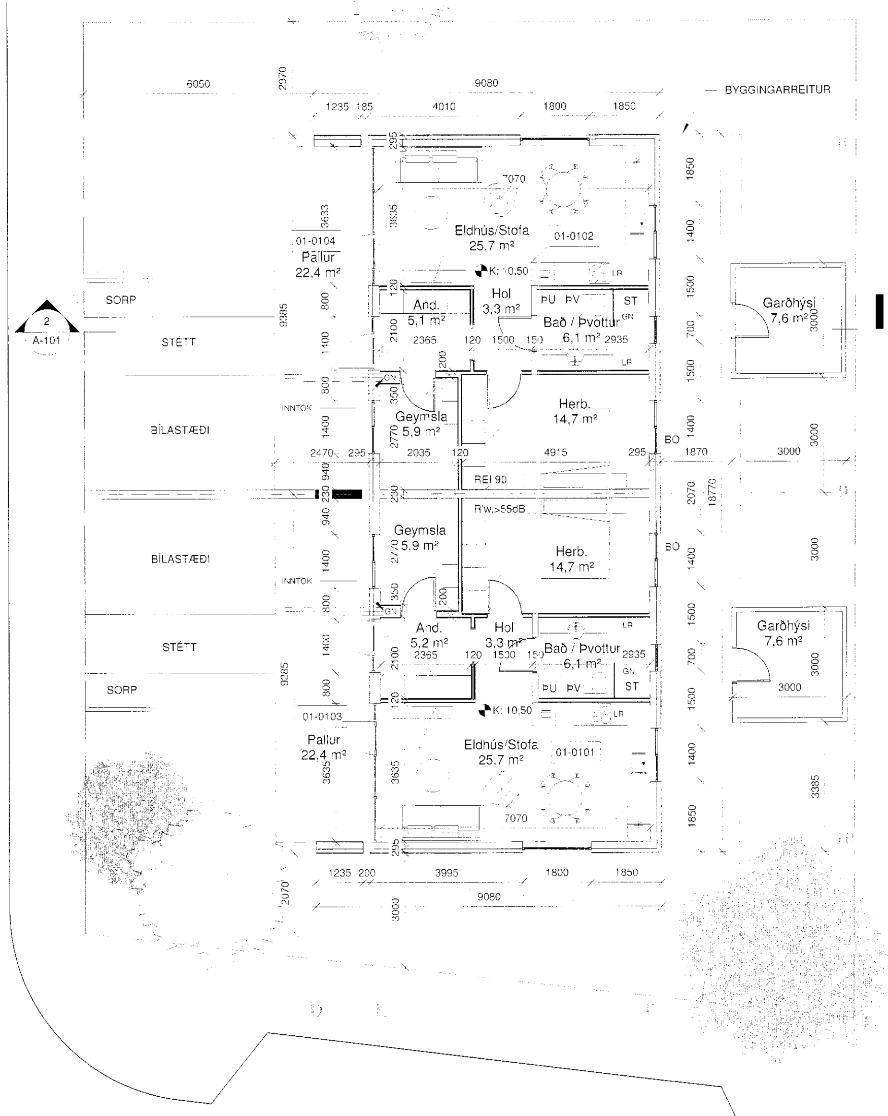
1 Grunnmynd 1 : 100
