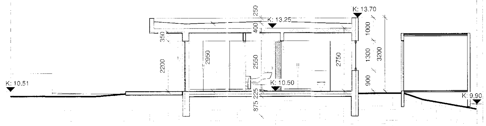
2 Snið A-A 1 : 100
