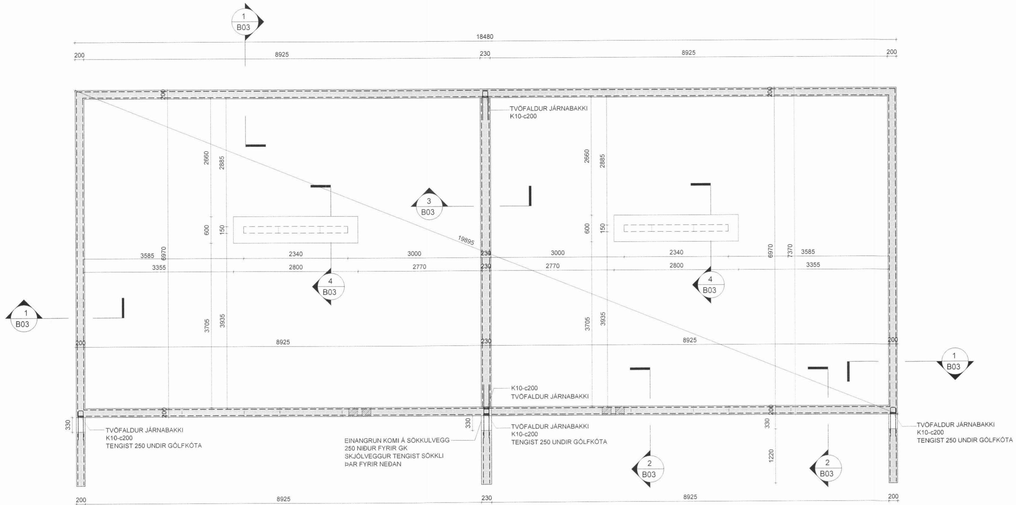
1 Grunnmynd sökkla 1 : 50
