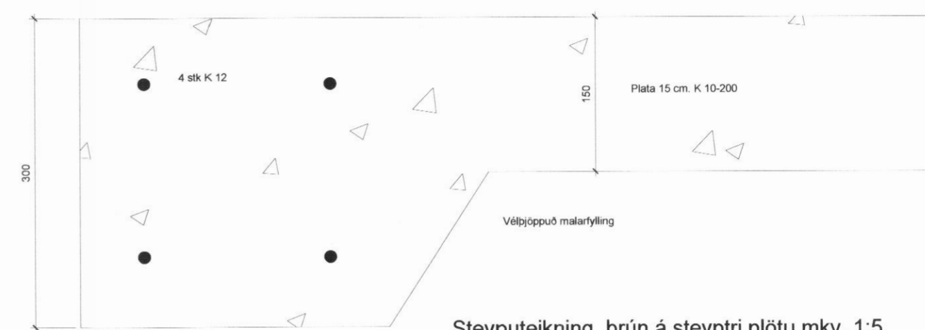
Steyputeikning, brún á steypri plötu mkv. 1:5
