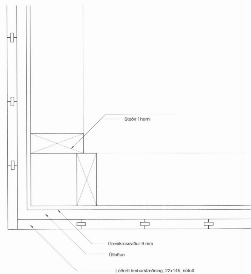
Þverskurður í gegnum horn
