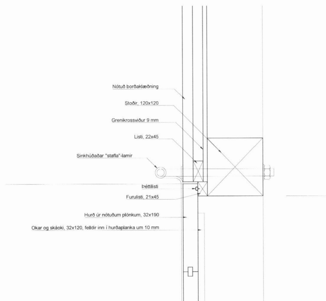
Þverskurður í gegnum gafflegg við bílskúrshurð
