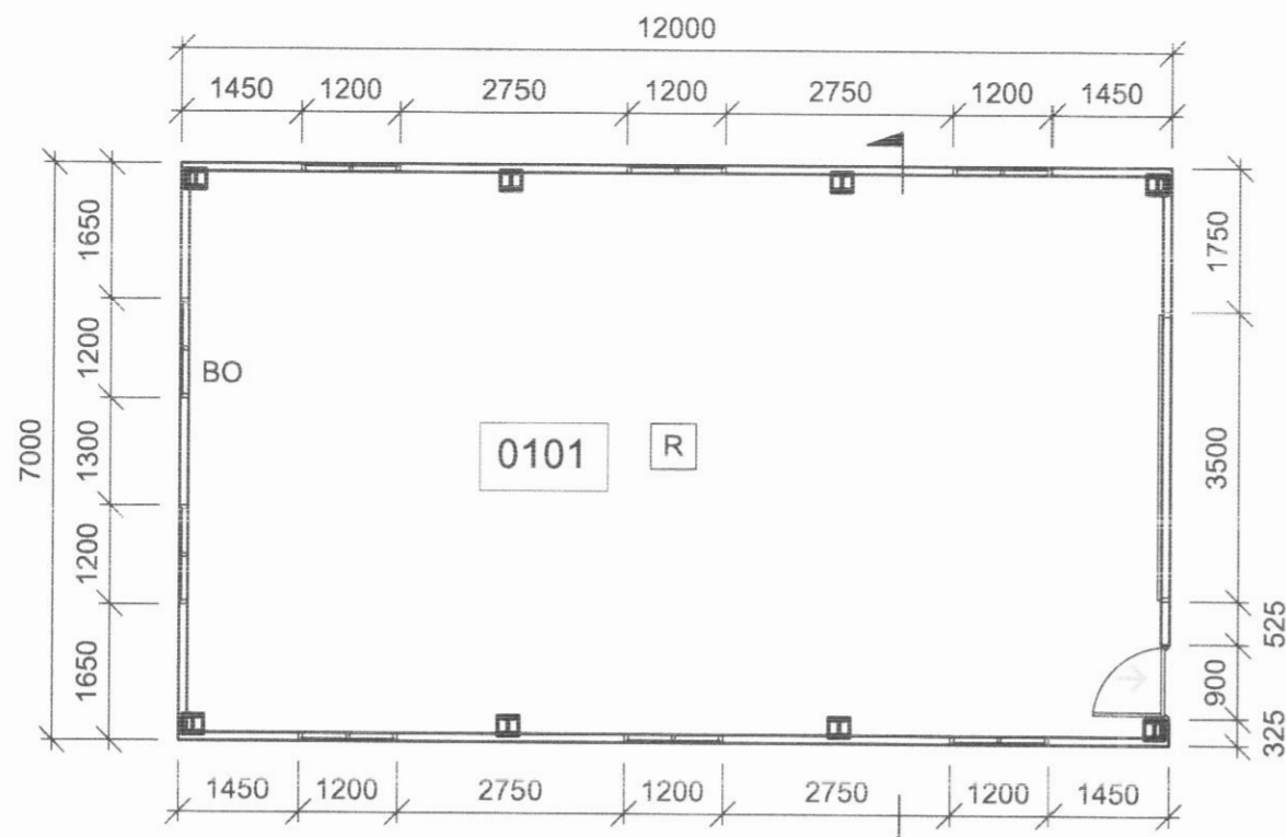
GRUNNMYND 1:100
