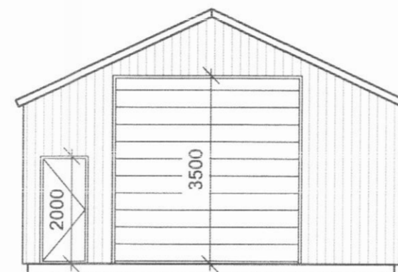
DYRSTAFN 1:100
