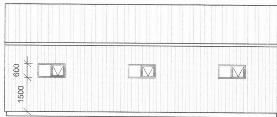
LANGHLÍÐ 1:100
