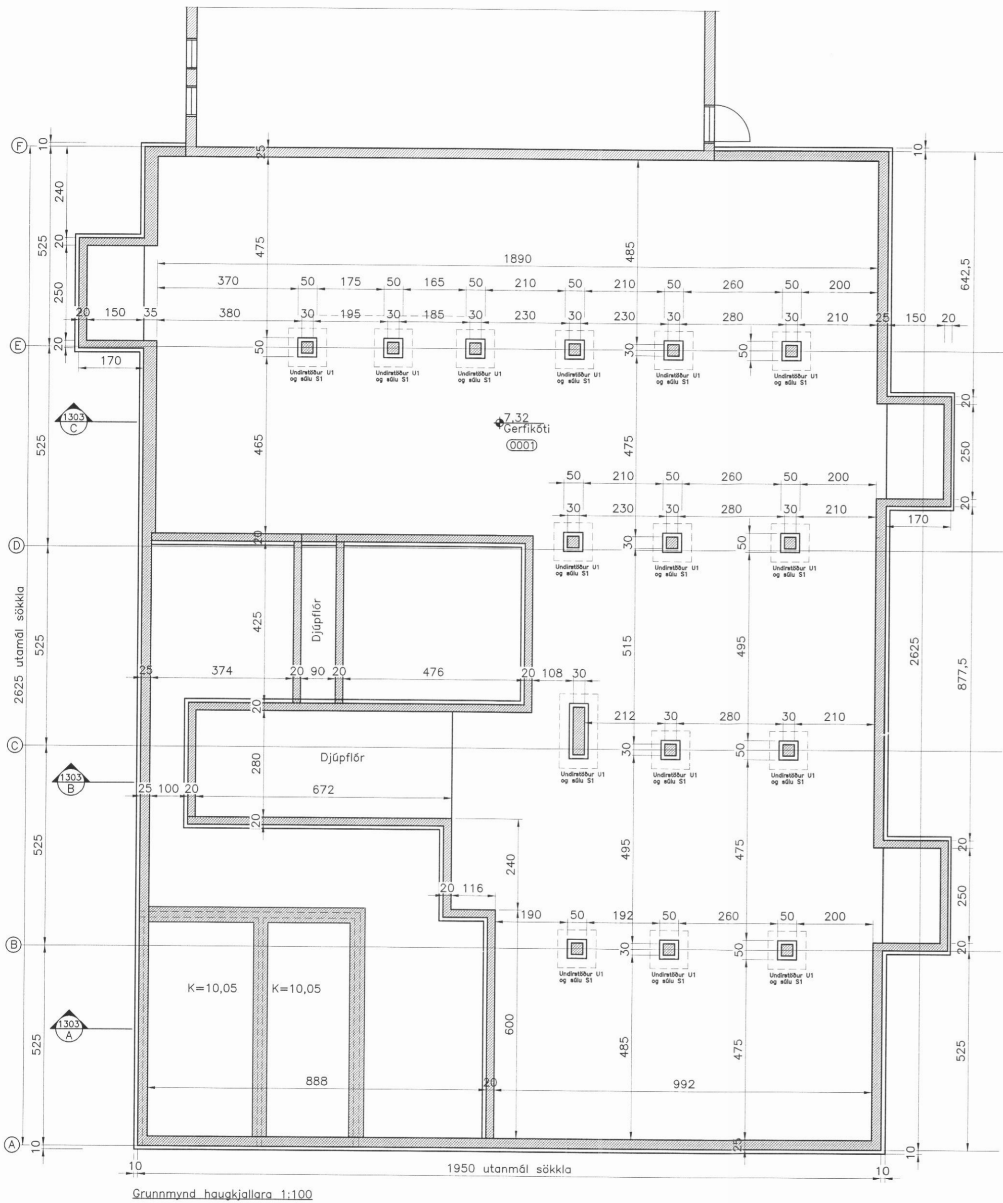
Grunnmynd haugkjallara 1:100
