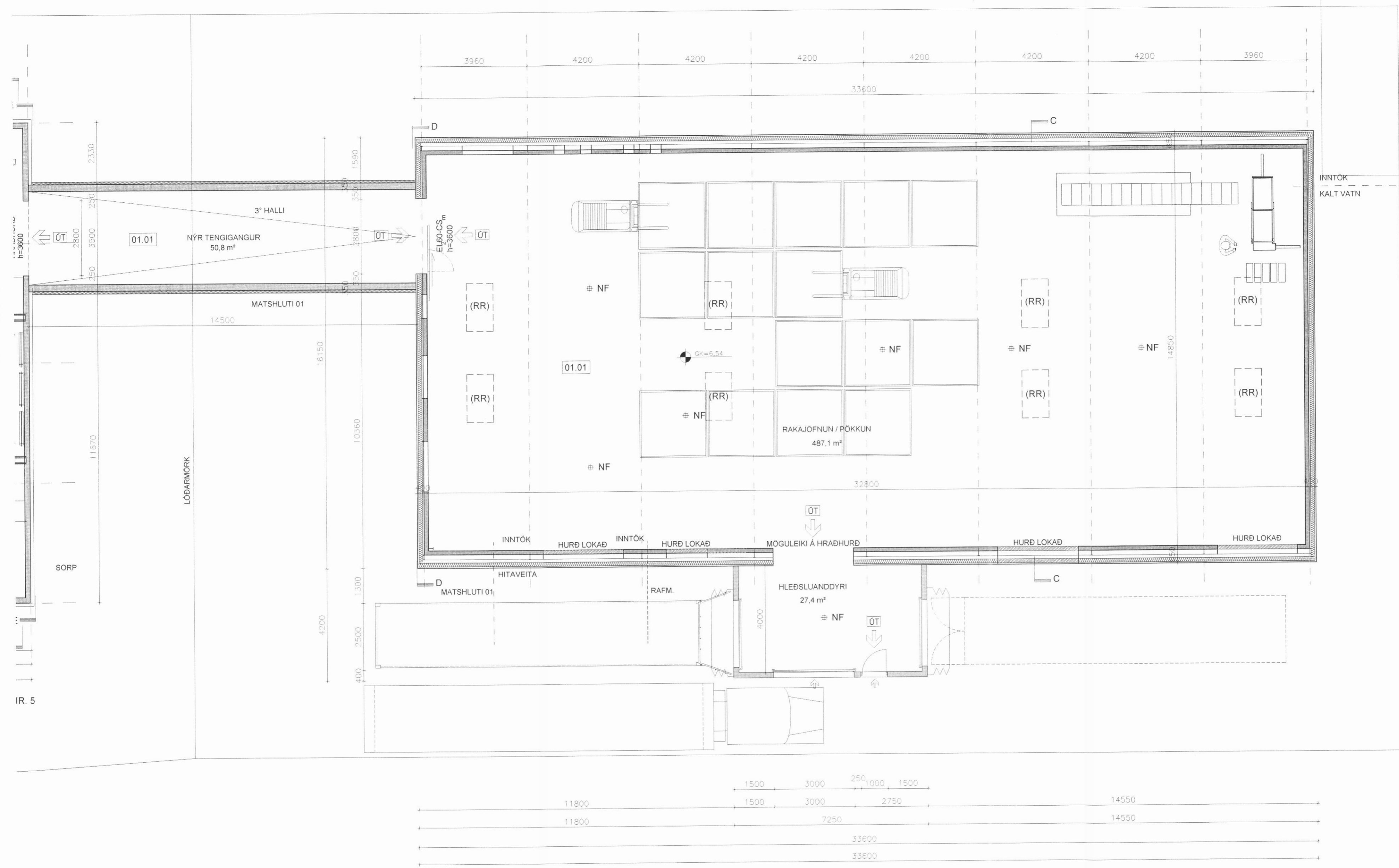
GRUNNMYND 1.HÆÐ MKV. 1:100
