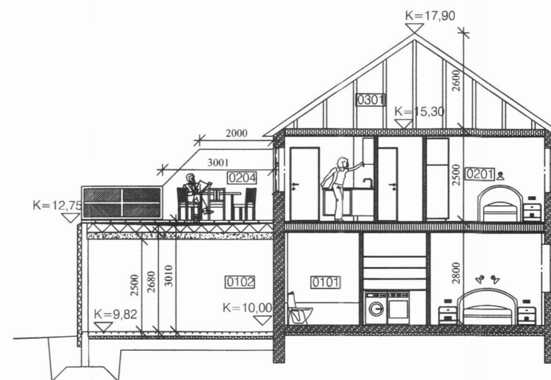
Sneiðmynd A:A 1:100
