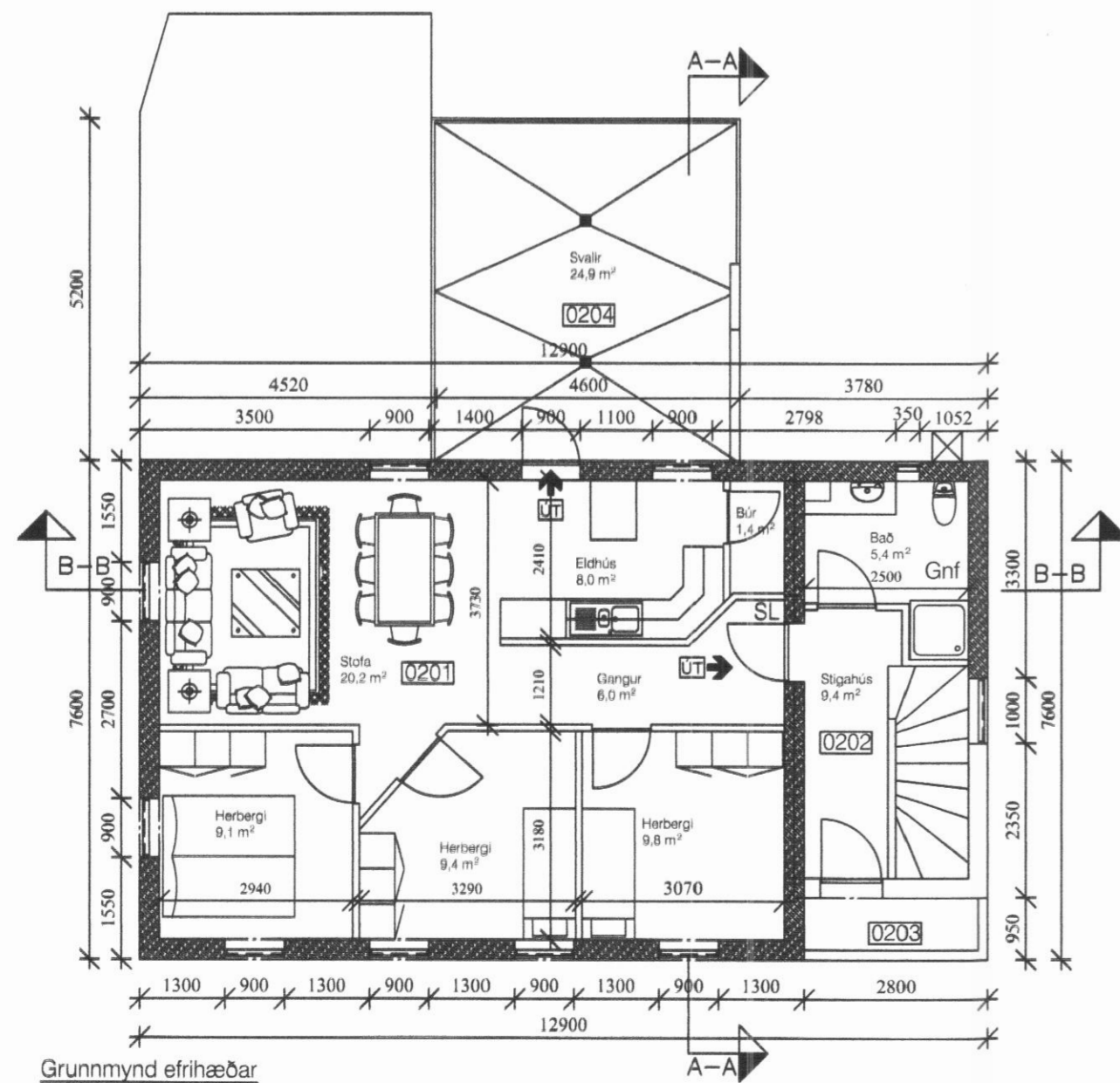
Grunnmynd efri hæðar 1:100
