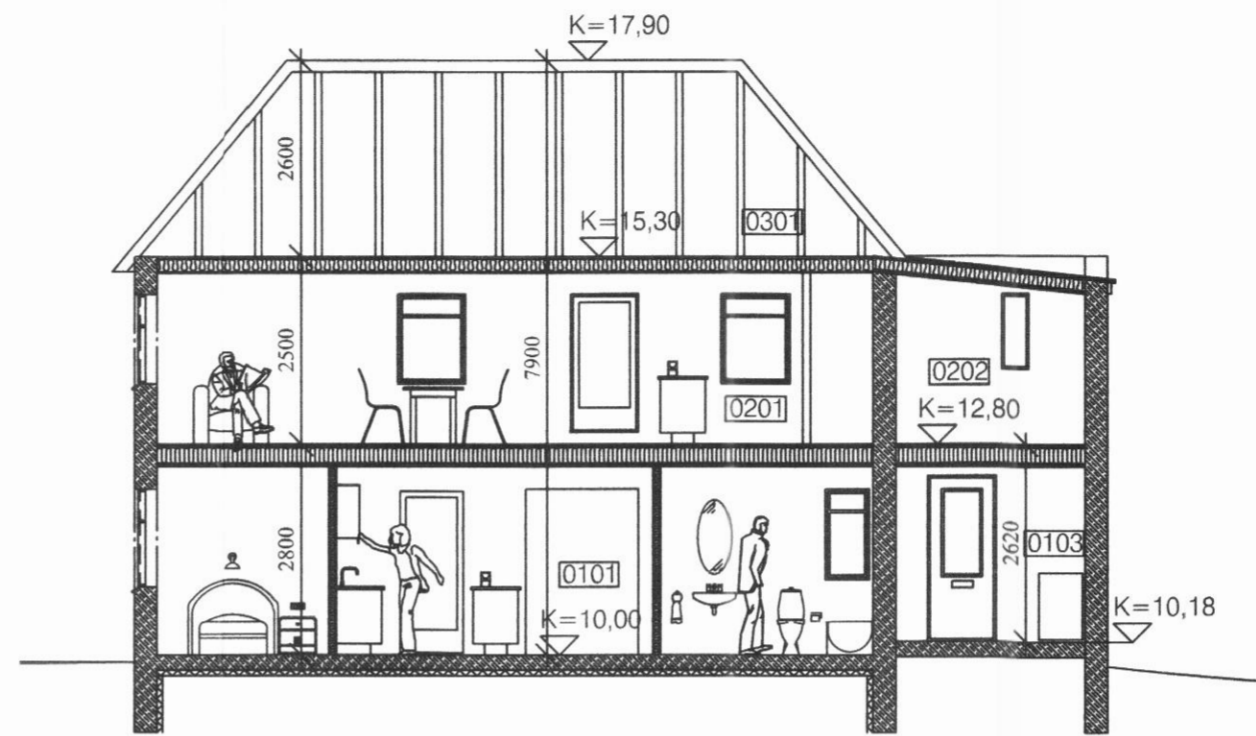
Sneiðmynd B:B 1:100
