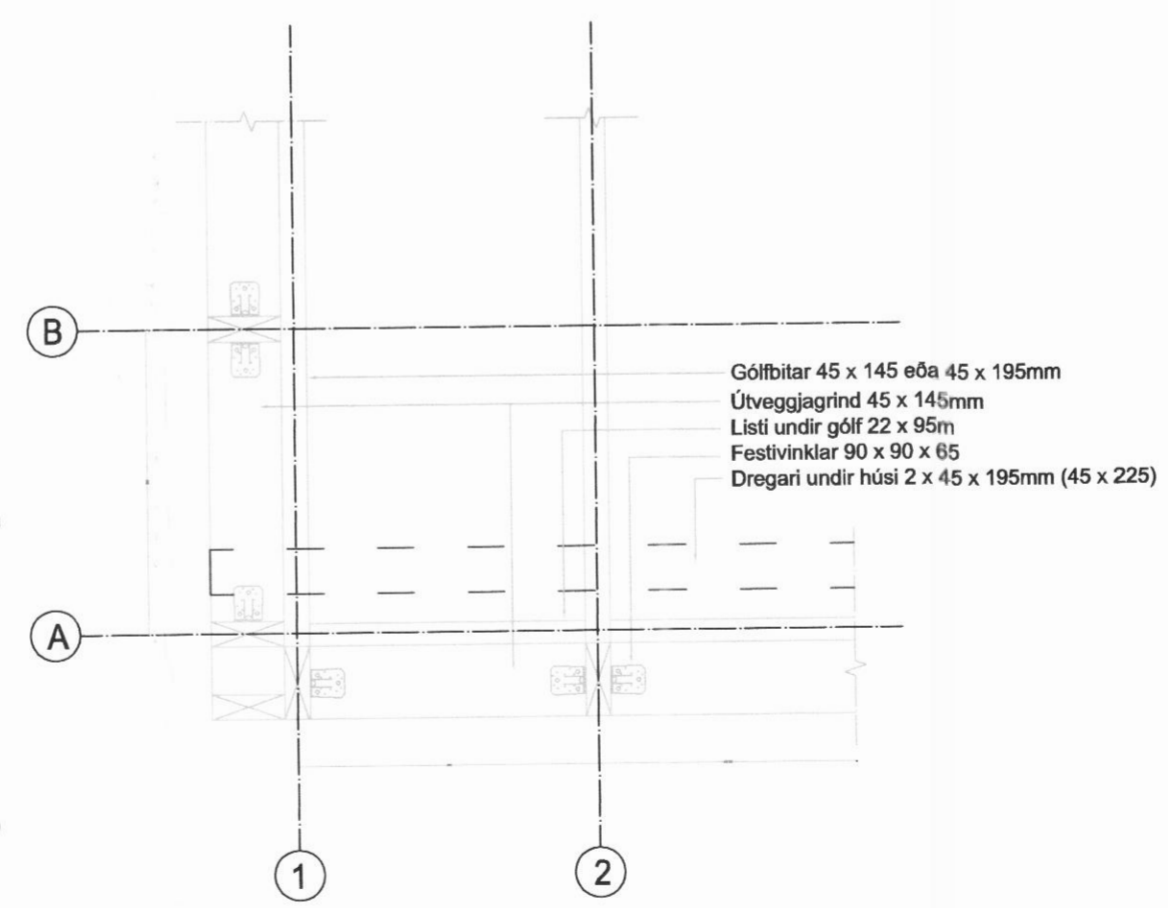
Grunnmynd: Lárétt mynd
