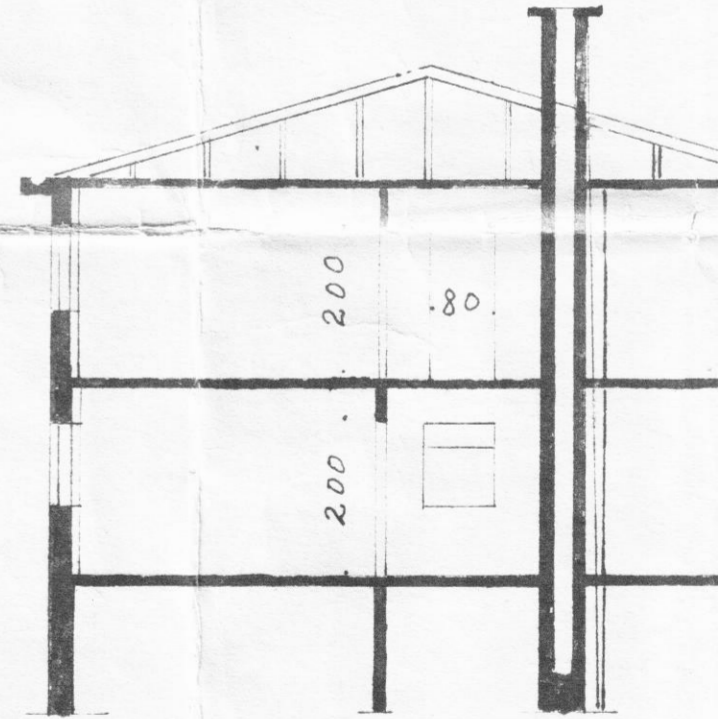
Þverskurður
