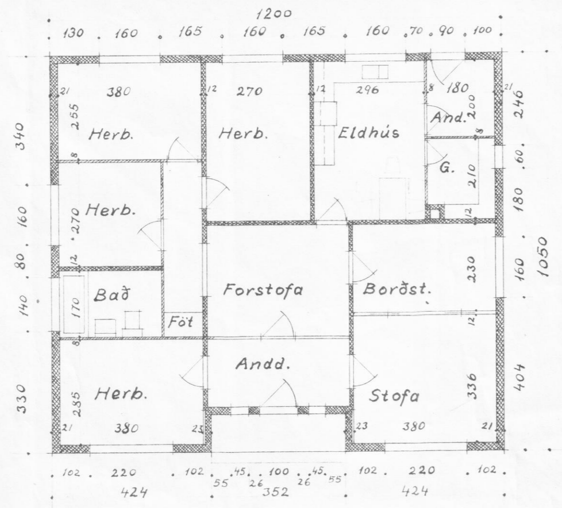
Grunnmynd
