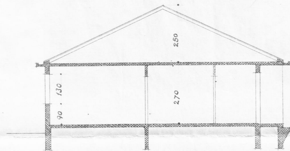
Skurður
