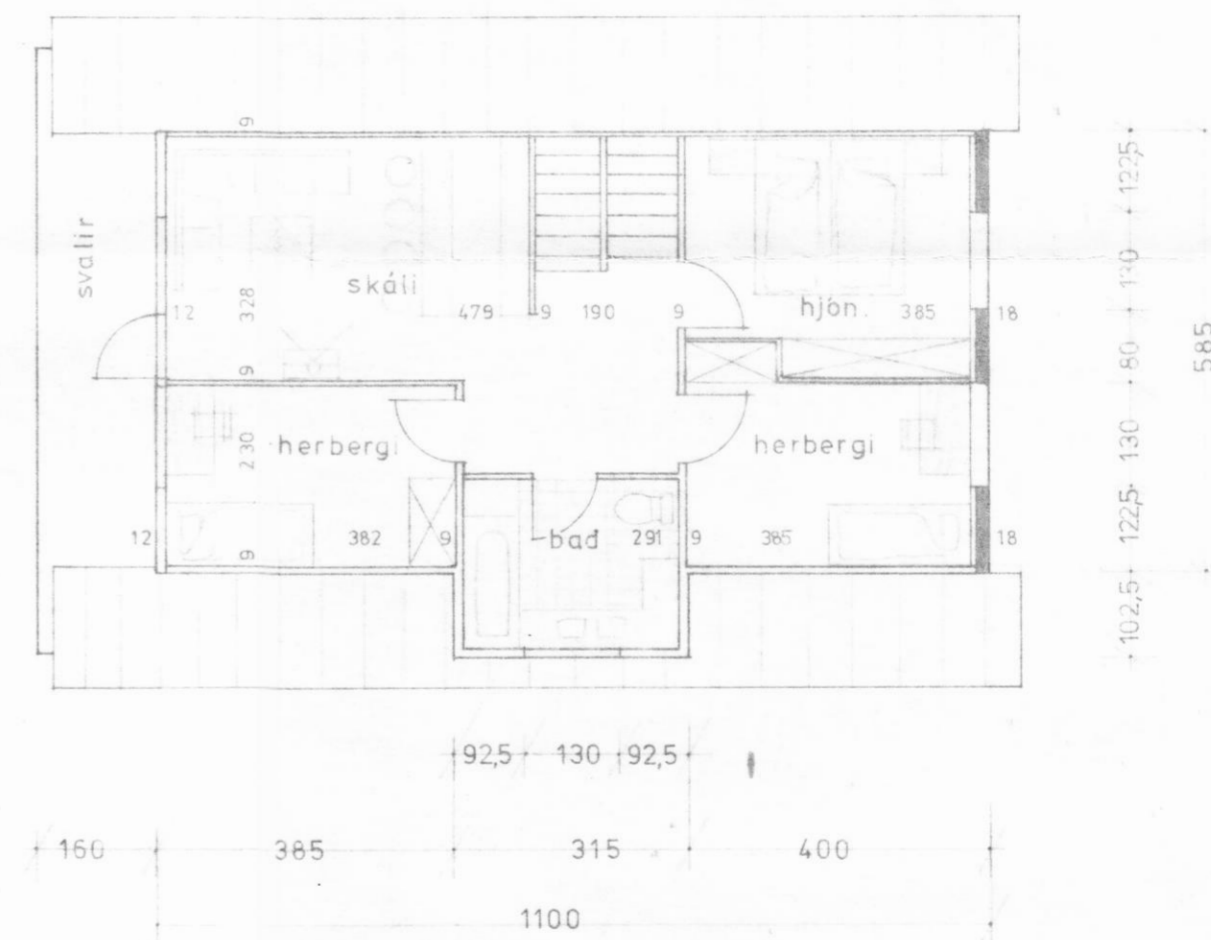
RISHÆÐ GRUNNMYND MKV. 1:100
