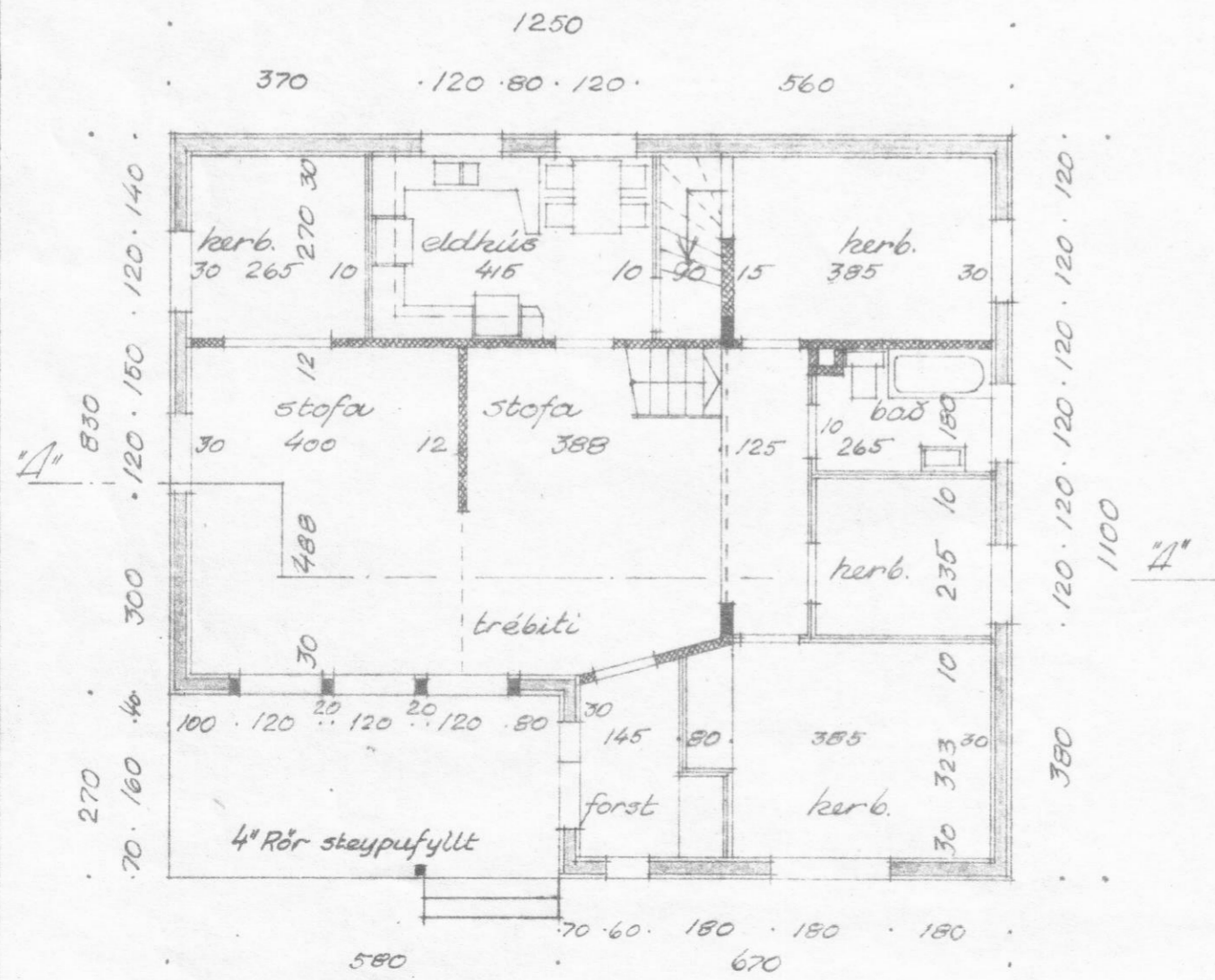
Mál 1:100
