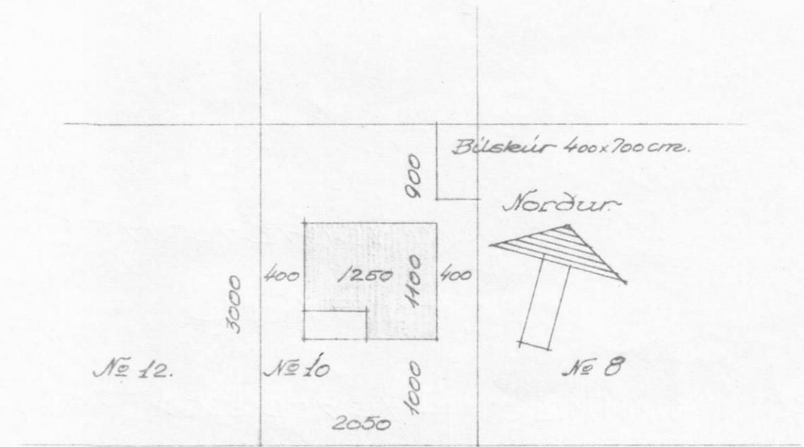
Godabyggð Mál 1:500
