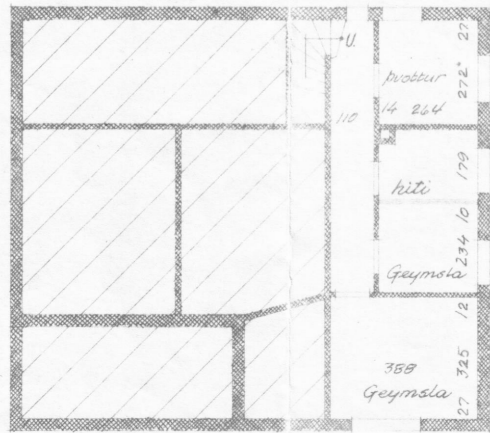
Mál 1:100
