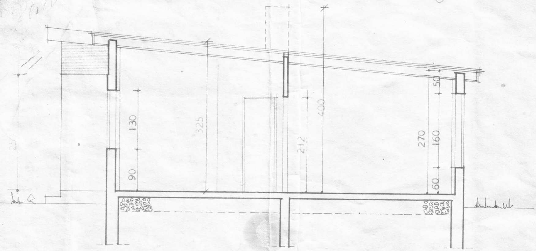
SNEIDING A--A
