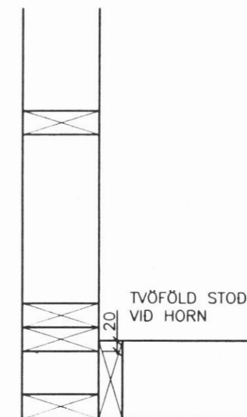
FRÁGANGUR VID HORN Mkv. 1:10
