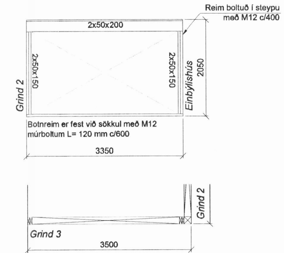
Grind 3 - Séð innanfrá MKV. 1:50
