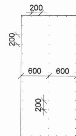
9mm Krossviðsplatá negld við stoðir með 200mm millibili
