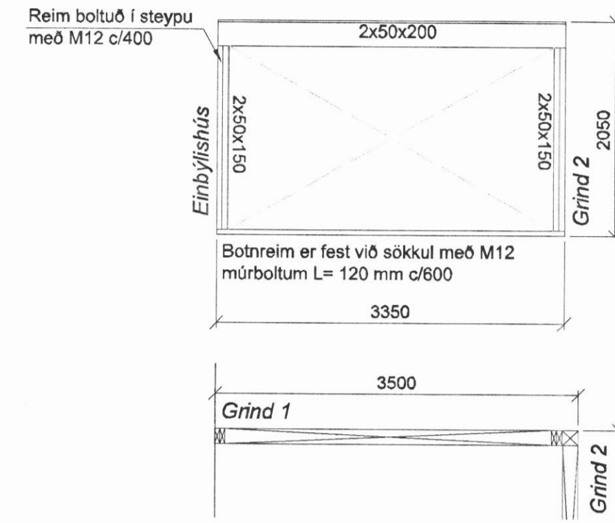
Grind 1 - Séð innanfrá MKV. 1:50
