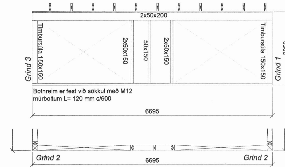
Grind 2 - Séð innanfrá MKV. 1:50
