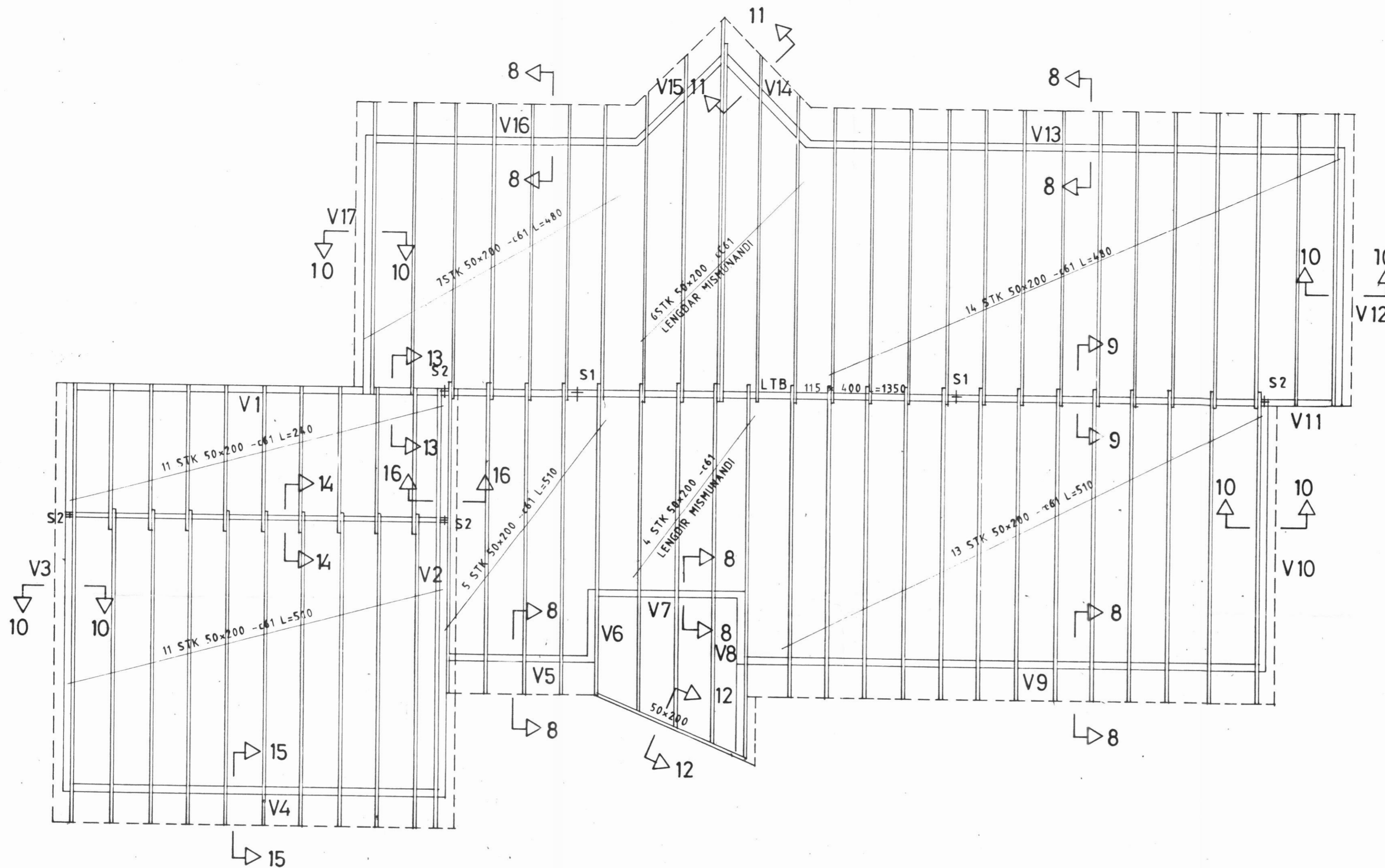
GRUNNMYND, 1:50
