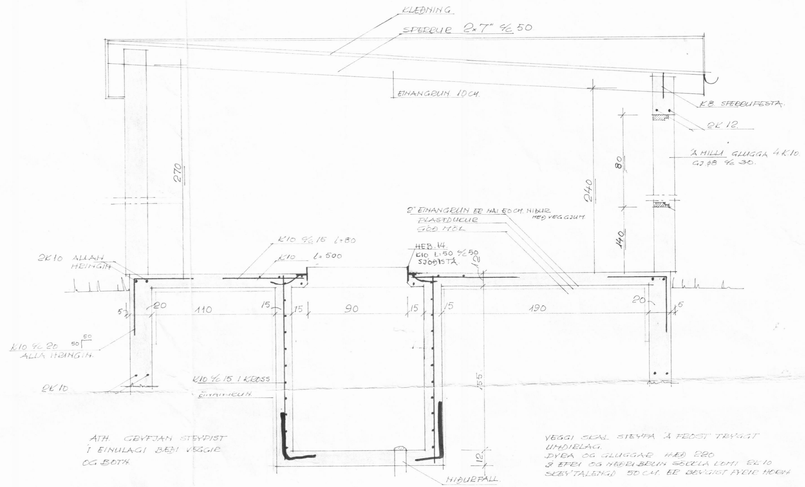
SNID A-A. M. 1:20
