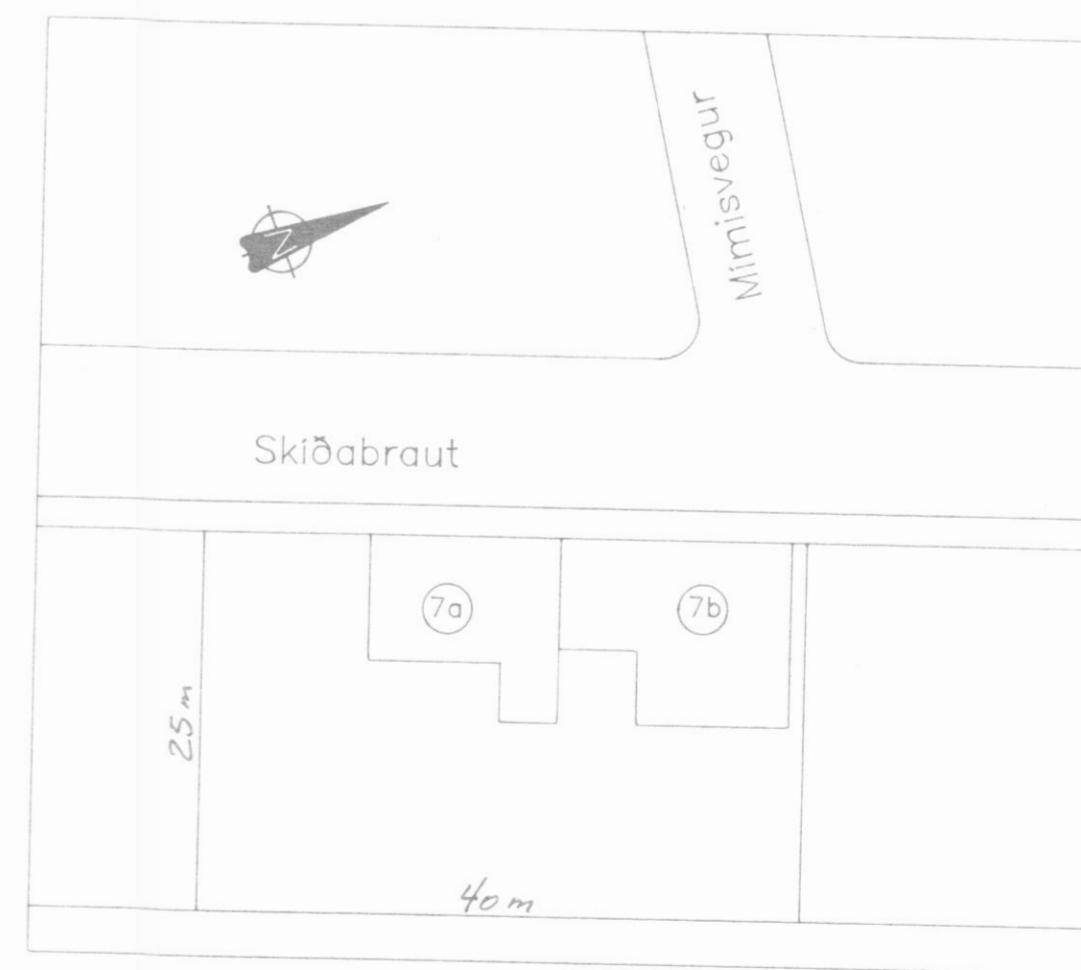
Afstöðumynd M 1:500
