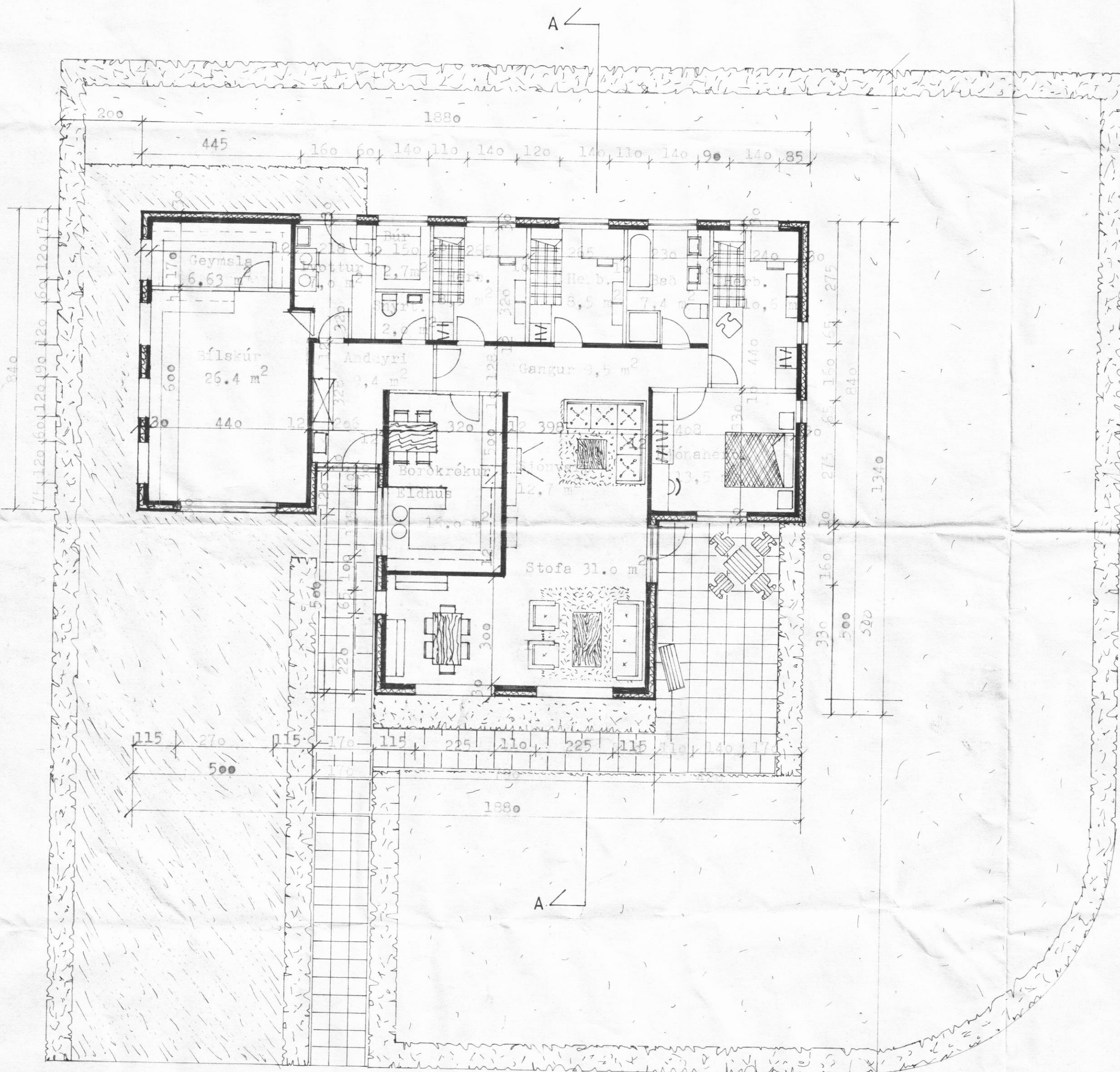
Grunnmynd, M=1:100.
