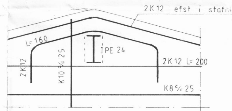
SN1Ð 3-3 Mkv. 1:20
