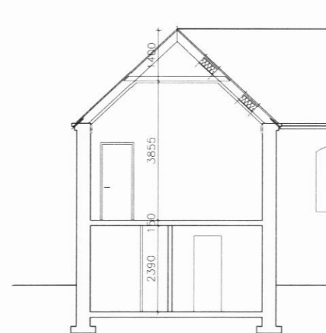
SNID C-C MKV. 1:100
