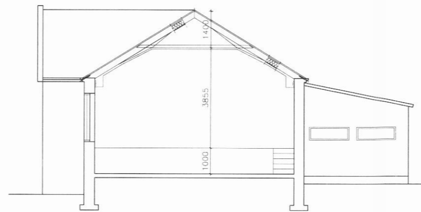
SNID A-A MKV. 1:100
