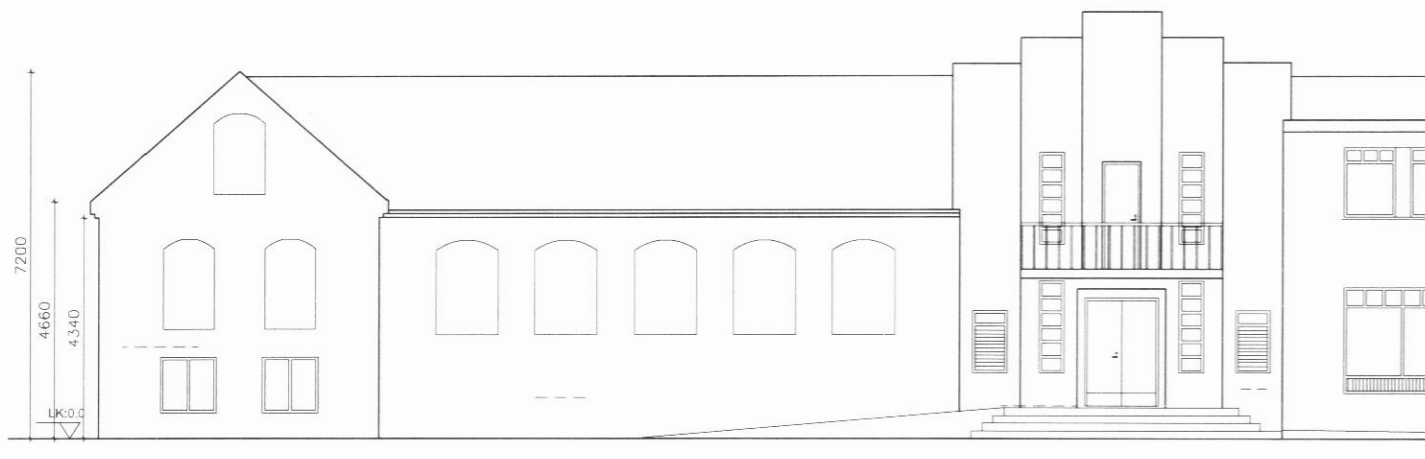
ÚTLIT UNGÓ, VESTUR MKV. 1:100
