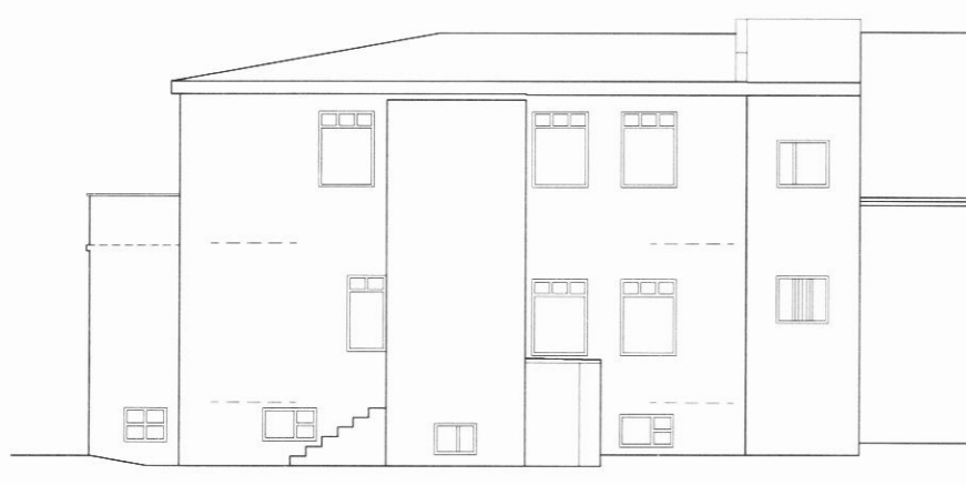
ÚTLIT SIGTÚN, AUSTUR MKV. 1:100
