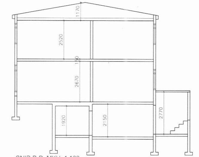
SNID B-B MKV. 1:100
