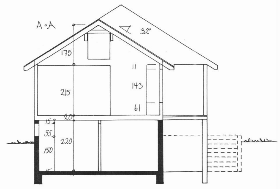
SNIÐ A-A
