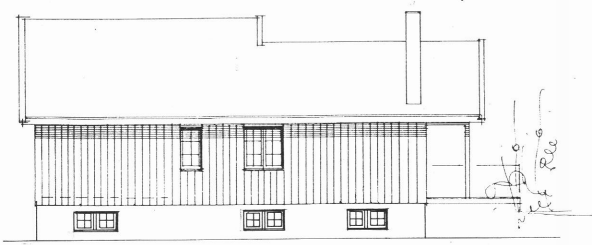
VESTURHLIÐ
