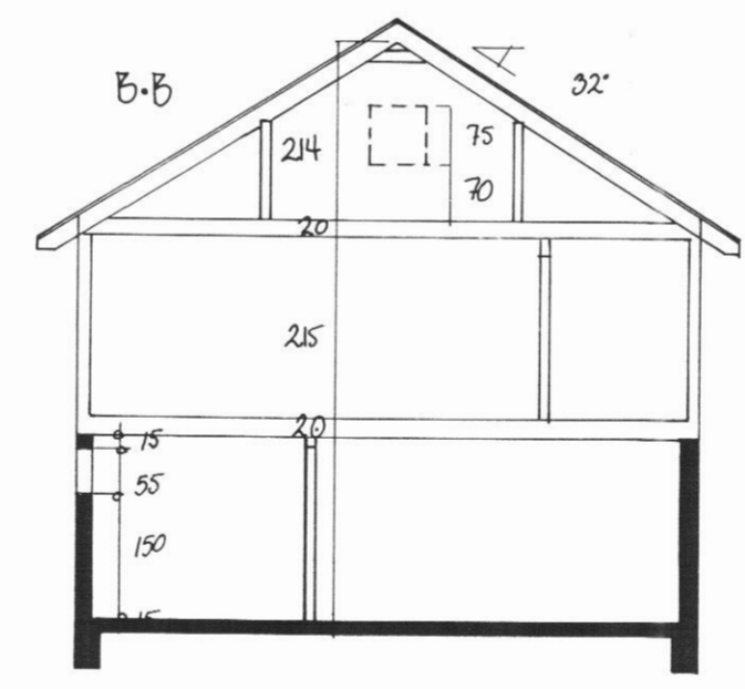
SNIÐ B-B
