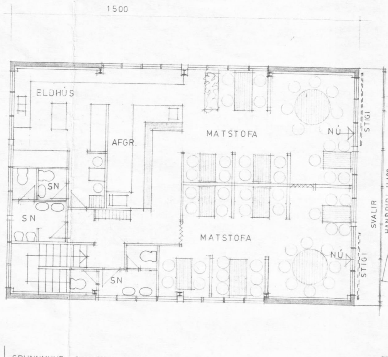
GRUNNMYND 2. HÆÐ
