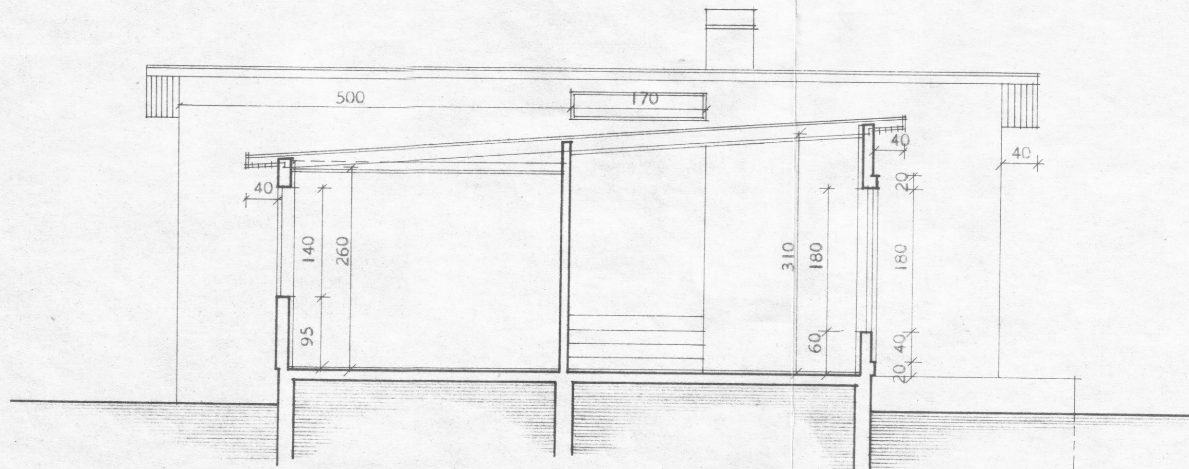
SNEIDING A - A
