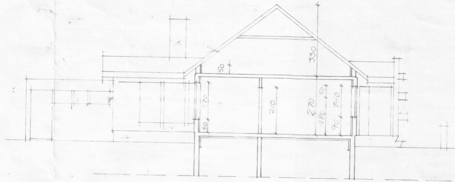
SNEIDING A-A
