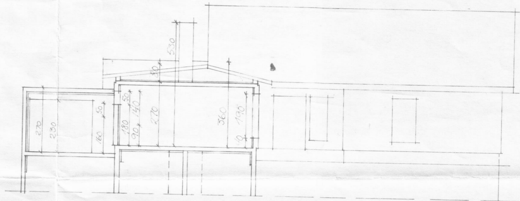
SNEIDING B-B
