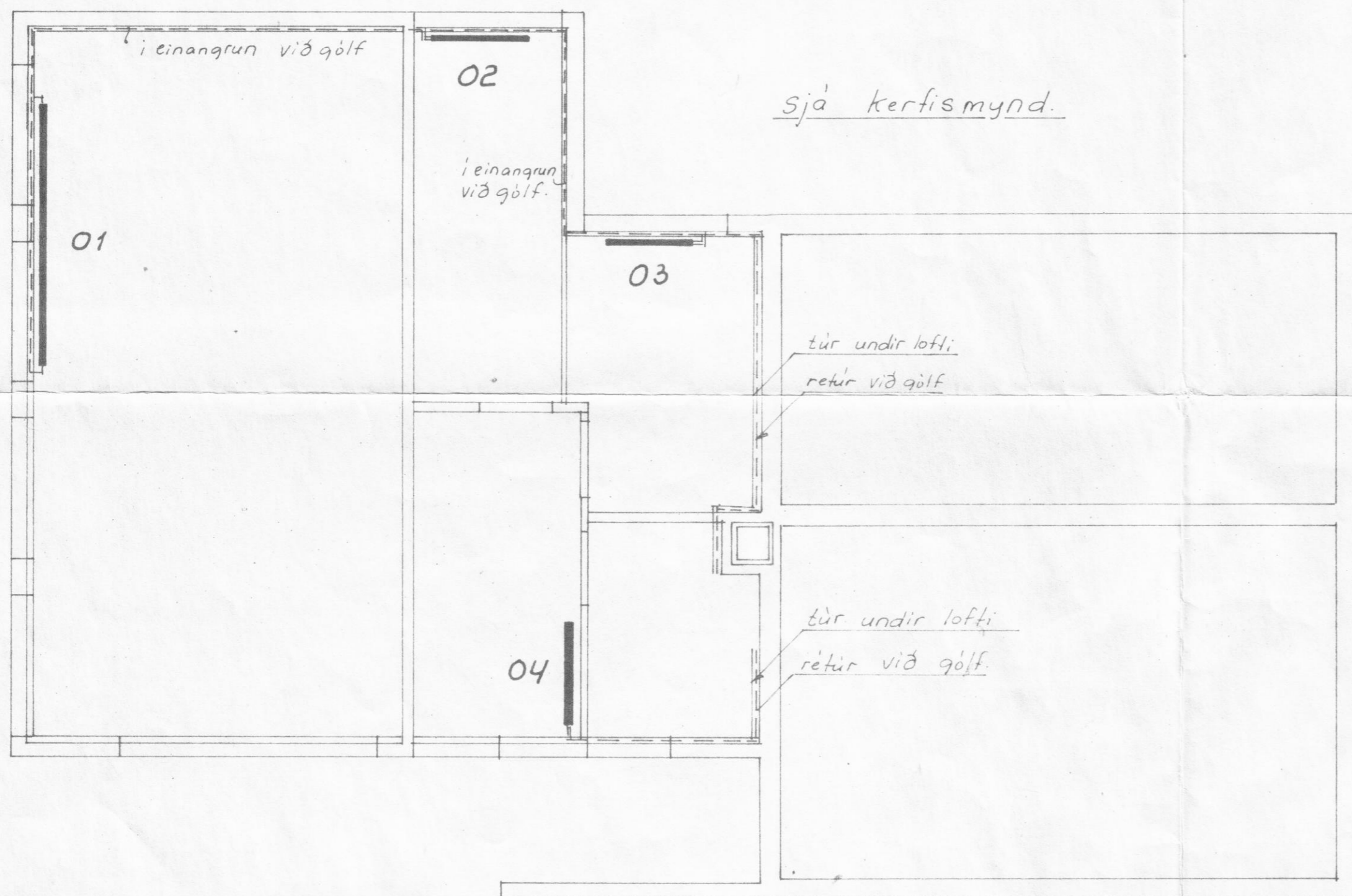
Grunnmynd kjallara 1:50
