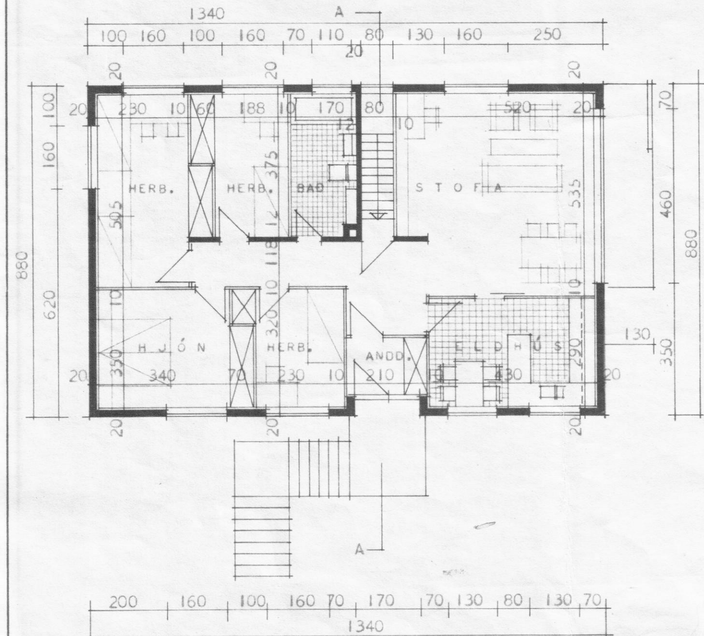
GRUNNMYND HEÐAR
