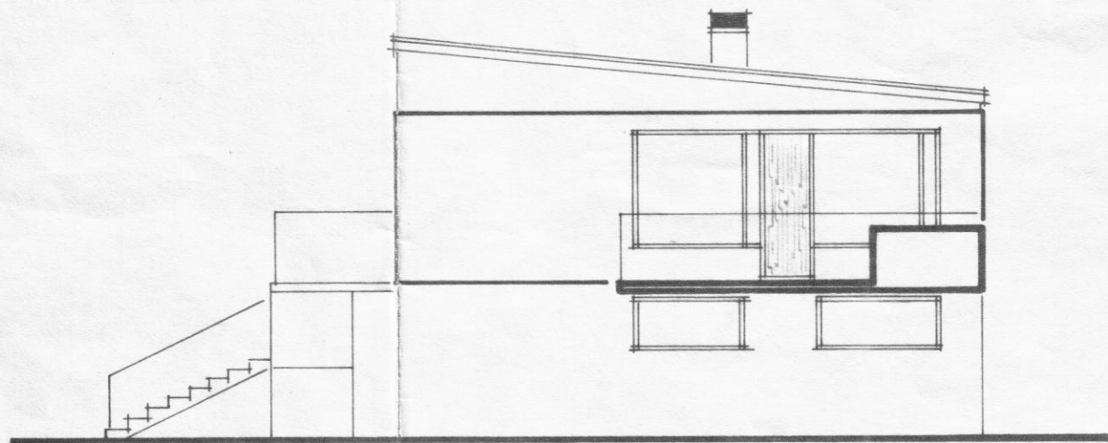
SUÐUR
