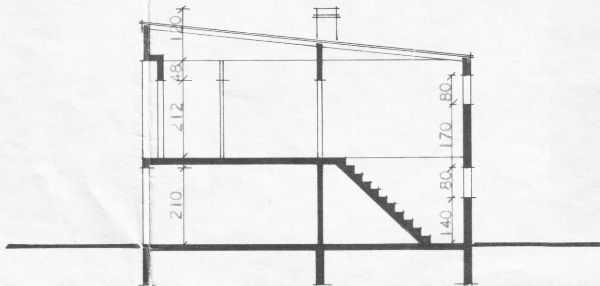
SNEIÐING A--A
