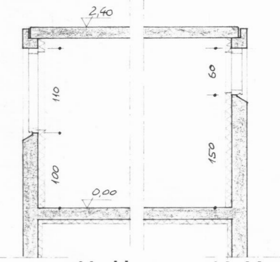
SKURÐUR u-u SKURÐUR v-v
