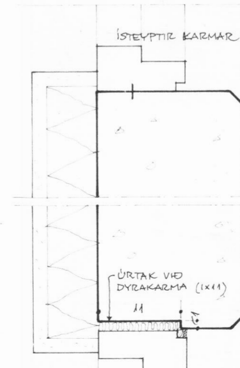
HLUTI H, 1:5
