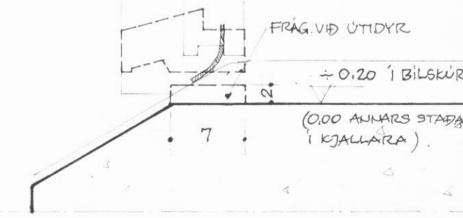
HLUTI G, 1:5
