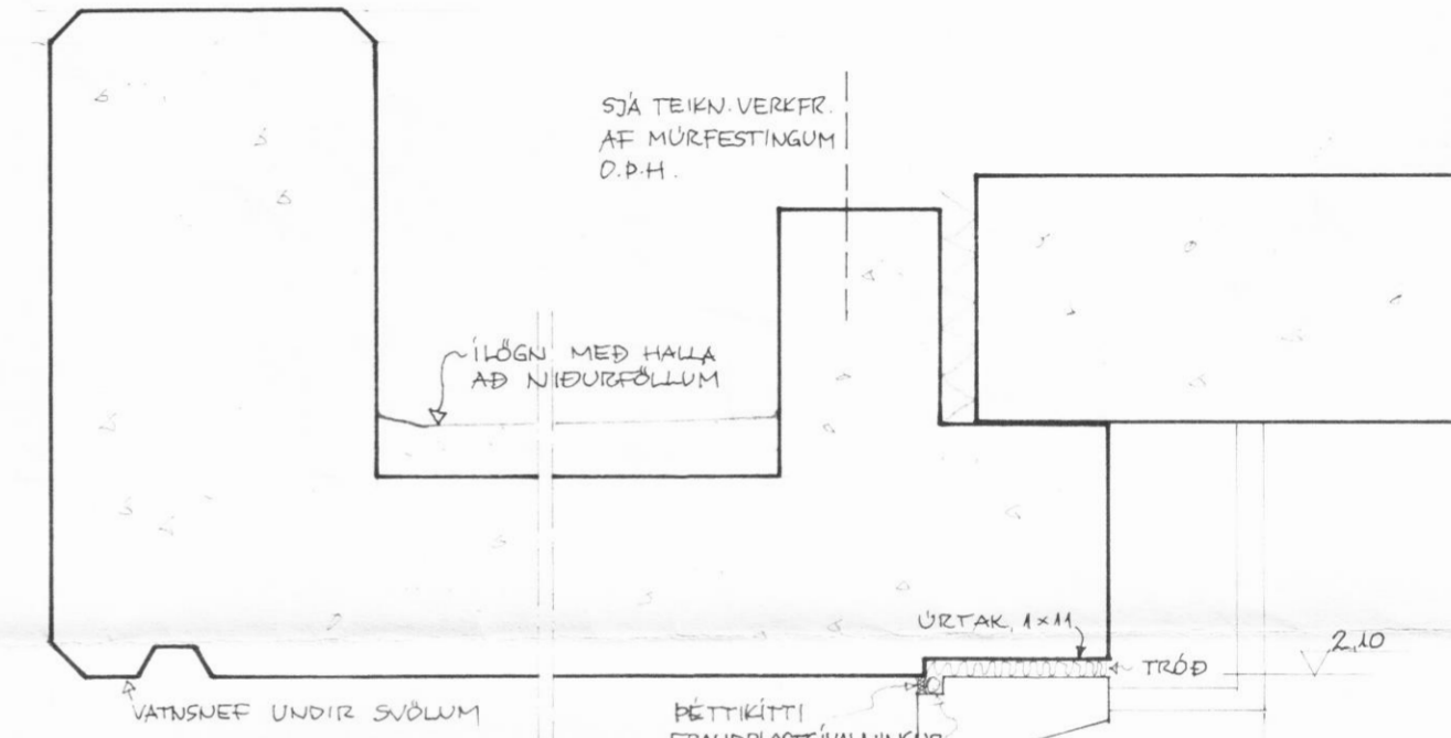
HLUTI E, 1:5
