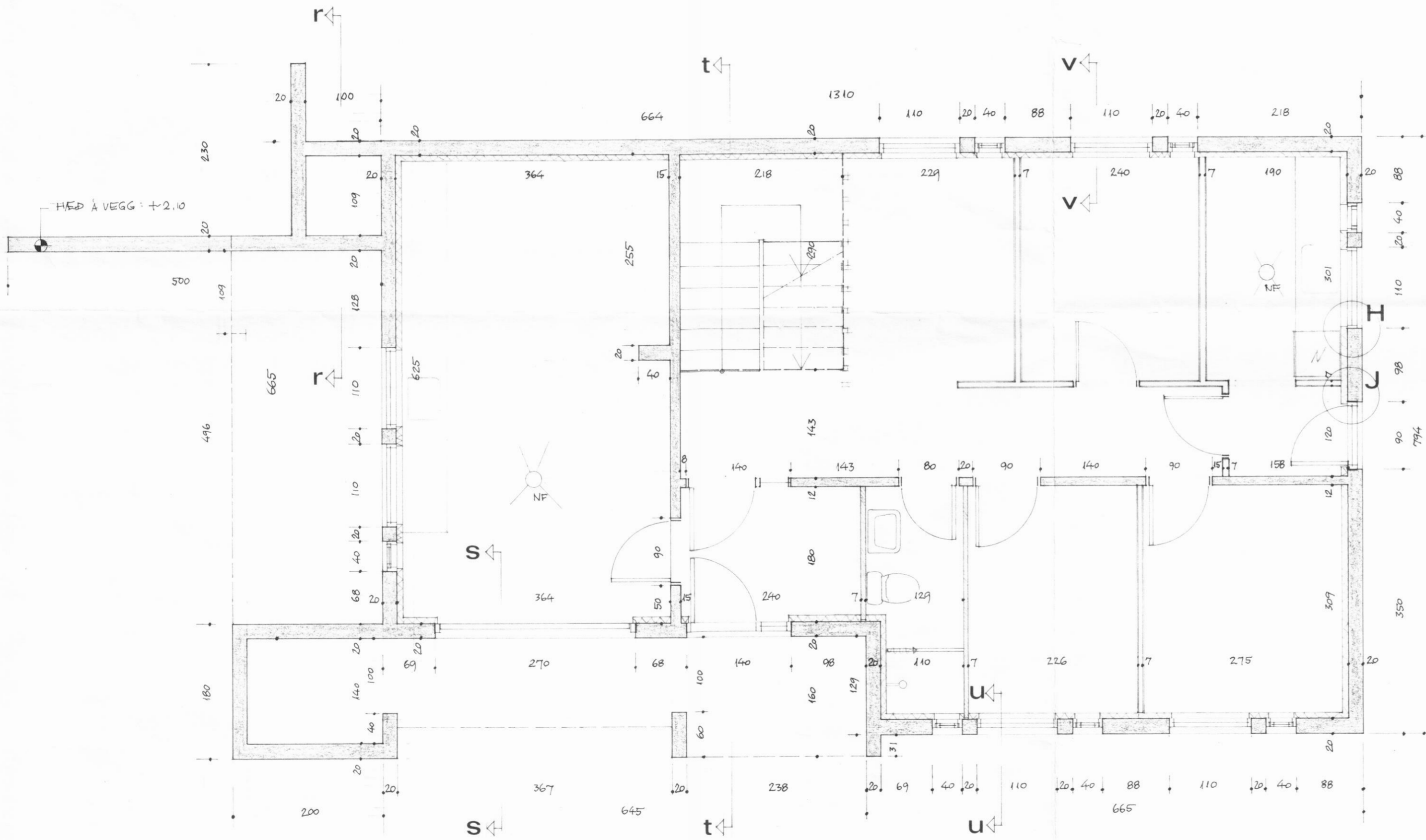
GRUNNMYND, 1:50
