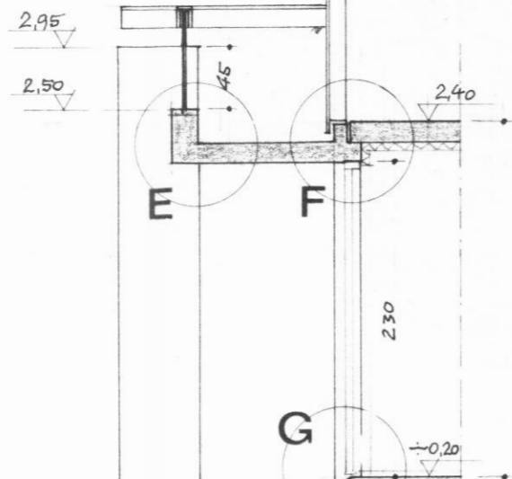
SKURÐUR s-s
