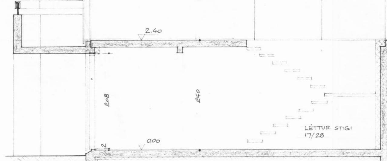
SKURÐUR t-t
