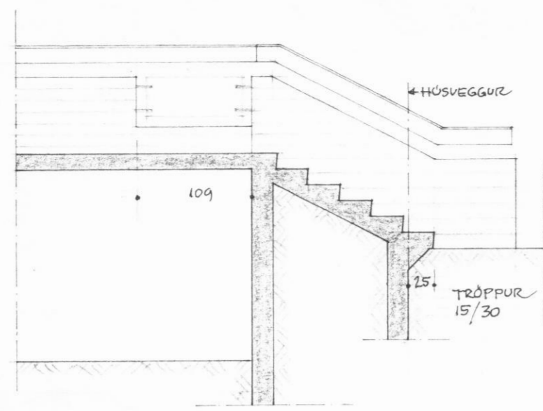
SKURÐUR r-r
