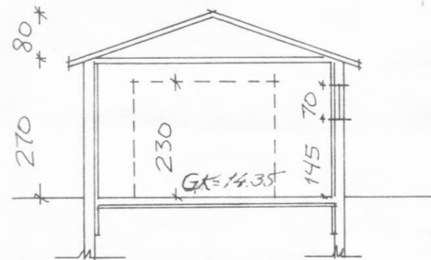
SNEIÐING 1:100
