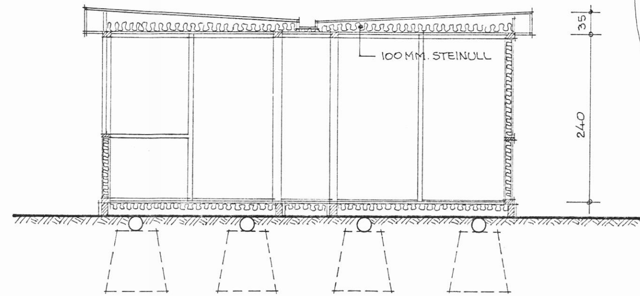
SNÍÐ
