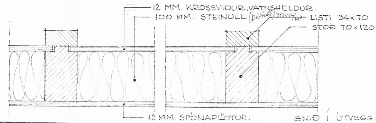
SNÍÐ
