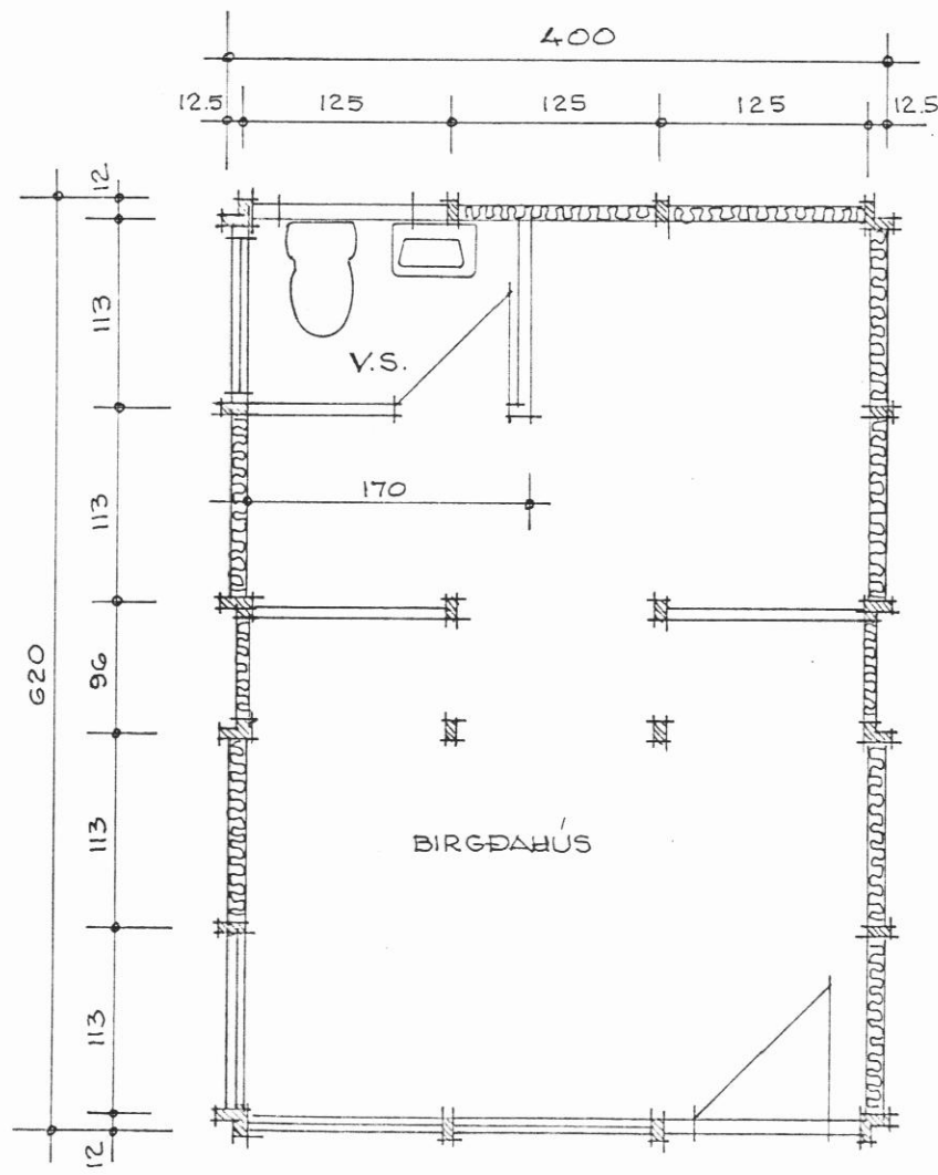
GRUNNMYND M = 1:50
