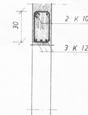
LÖÐR. SNID 1:20
