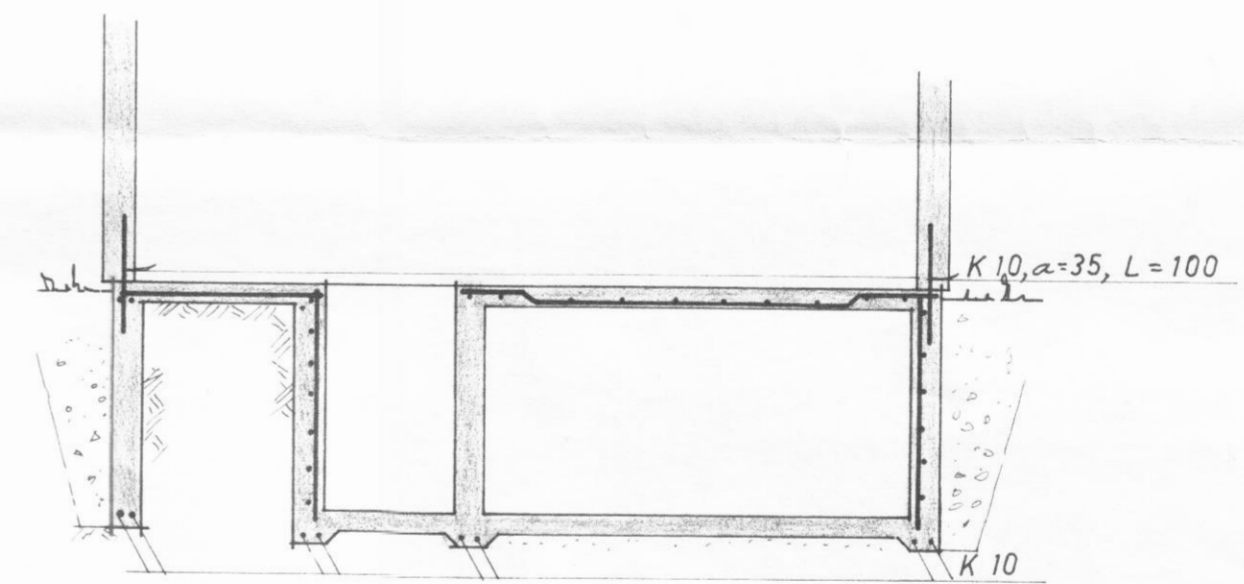
SNID A-A 1:50
