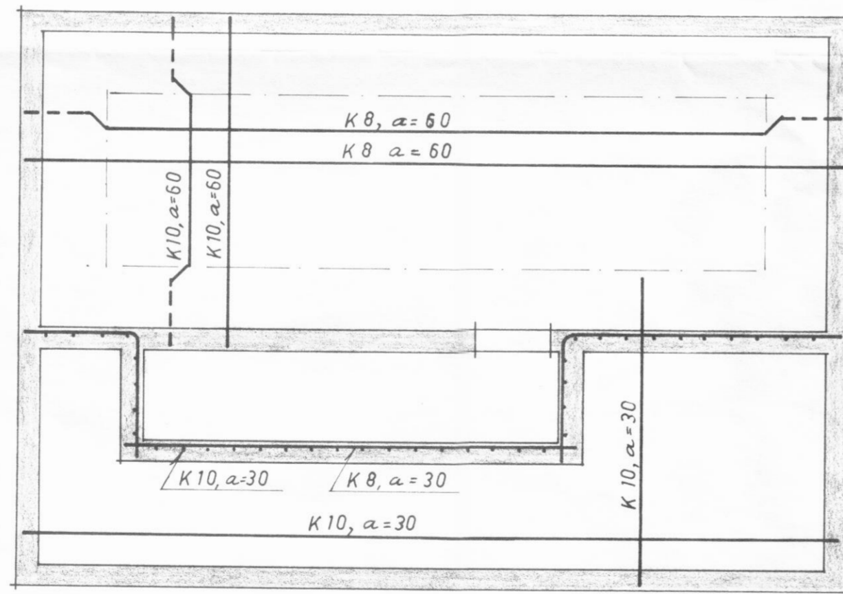
GÖLFPLATA 1:50
