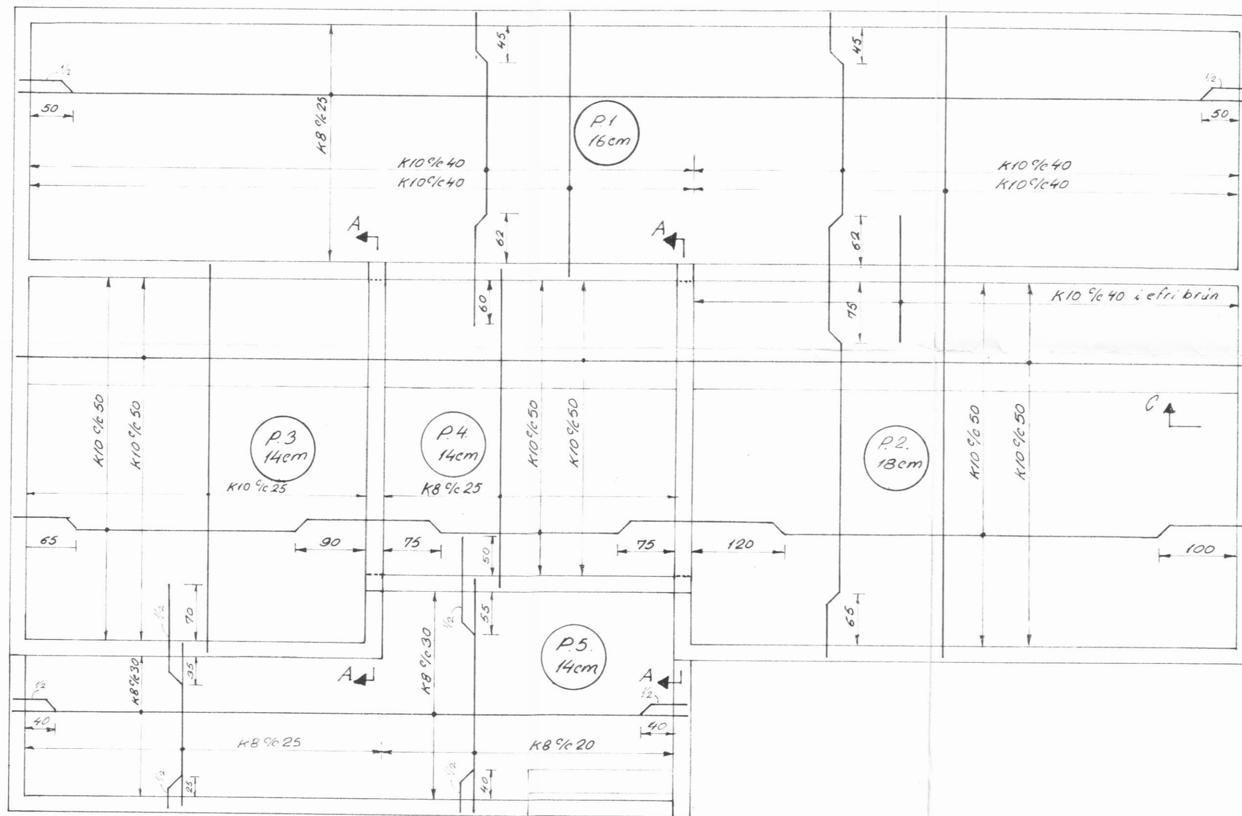
Plan af gölfplötu, jörnbending 1:50
